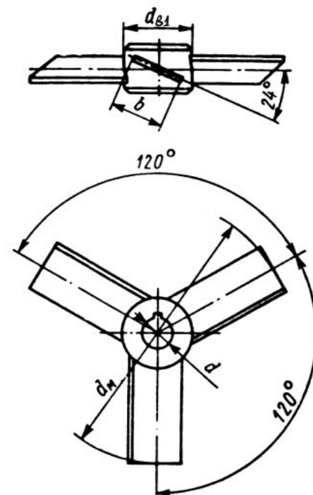
а - трехлопастная мешалка;
