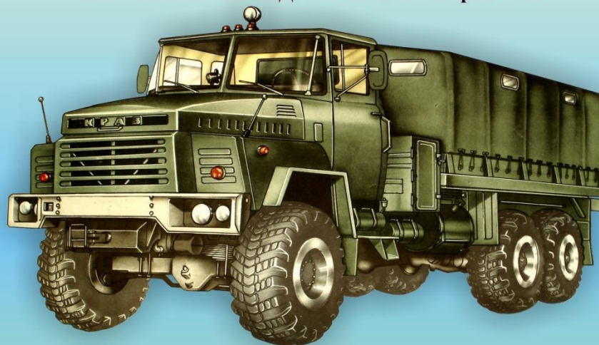
ЗАГАЛЬНИЙ ВИГЛЯД АВТОМОБІЛЯ КрАЗ-6322
