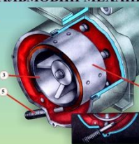
ГАЛЬМОВИЙ МЕХАНІЗМ
