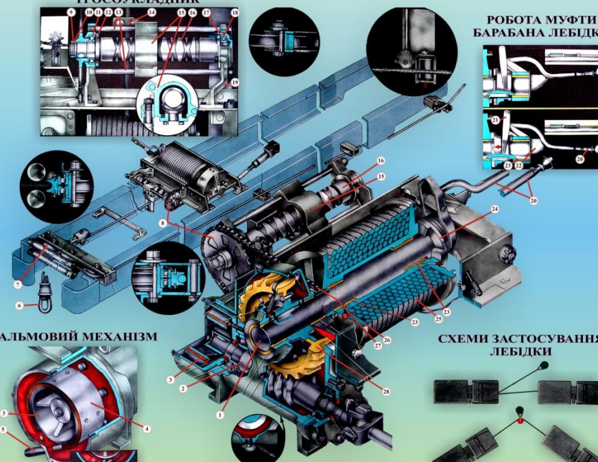
ТРОСОУКЛАДНИК
