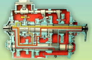
ПРИВІД УПРАВЛІННЯ КОРІБКОЮ ПЕРЕДАЧ
