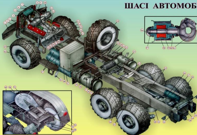
ШАСІ АВТОМОБІЛЯ КрАЗ-6322
