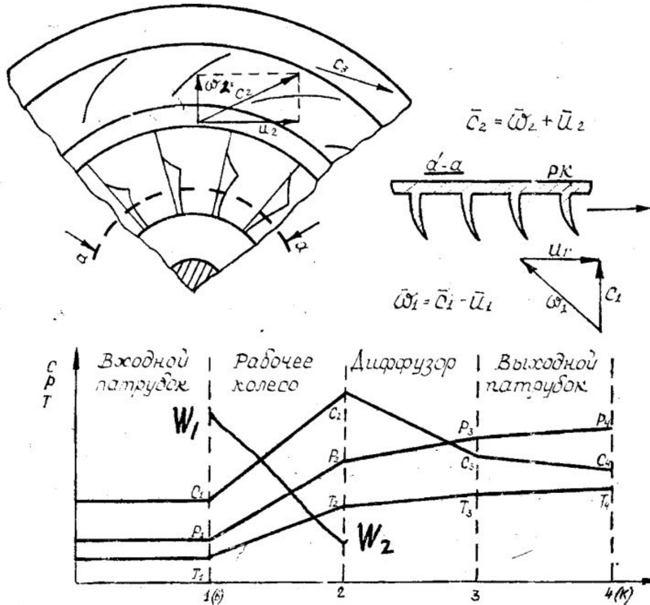
Рис.1.1 Изменение параметров потоков воздуха в центробежном компрессоре
