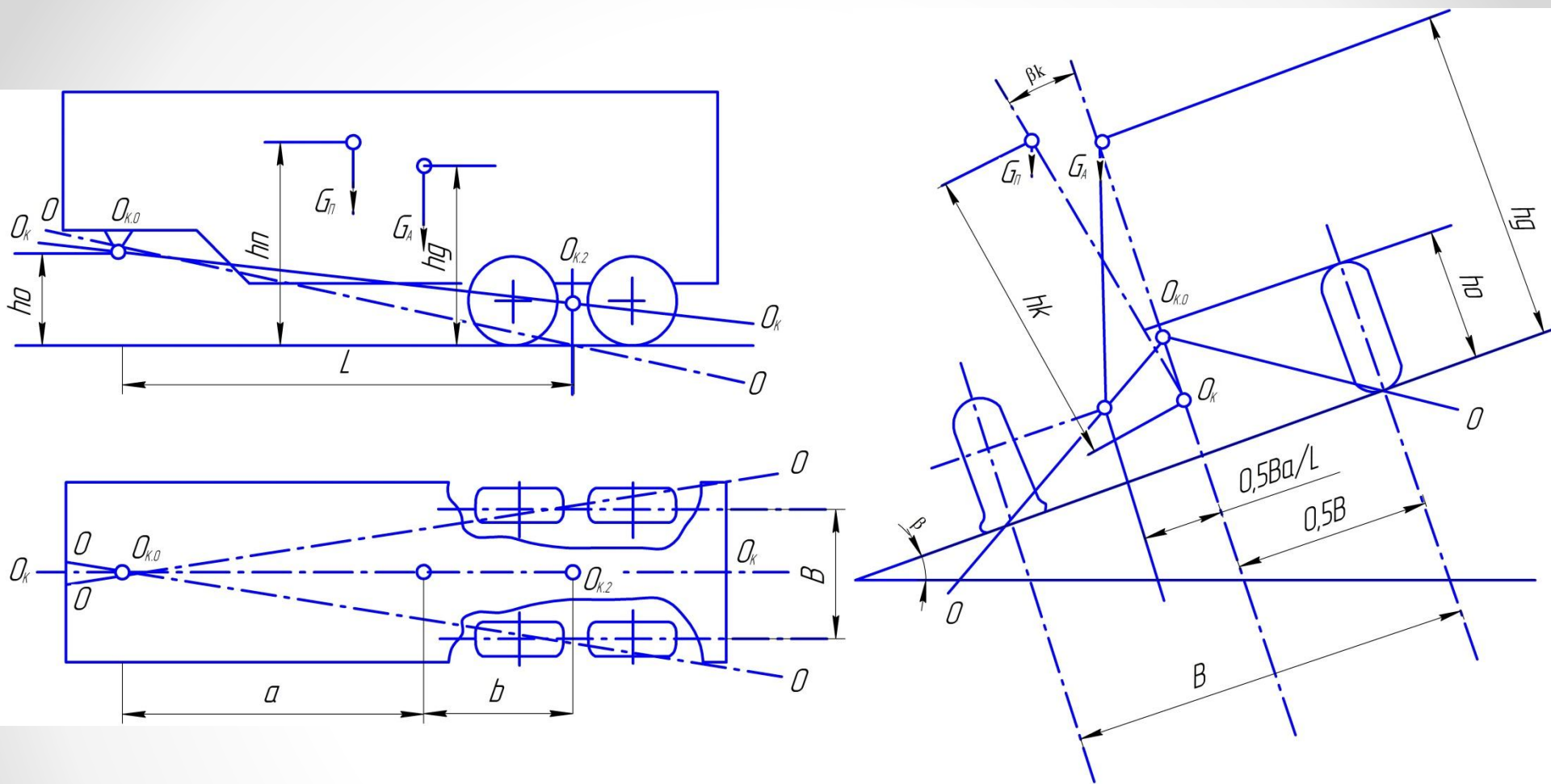
Рис.2. Розрахункова модель А.М. Петренко
