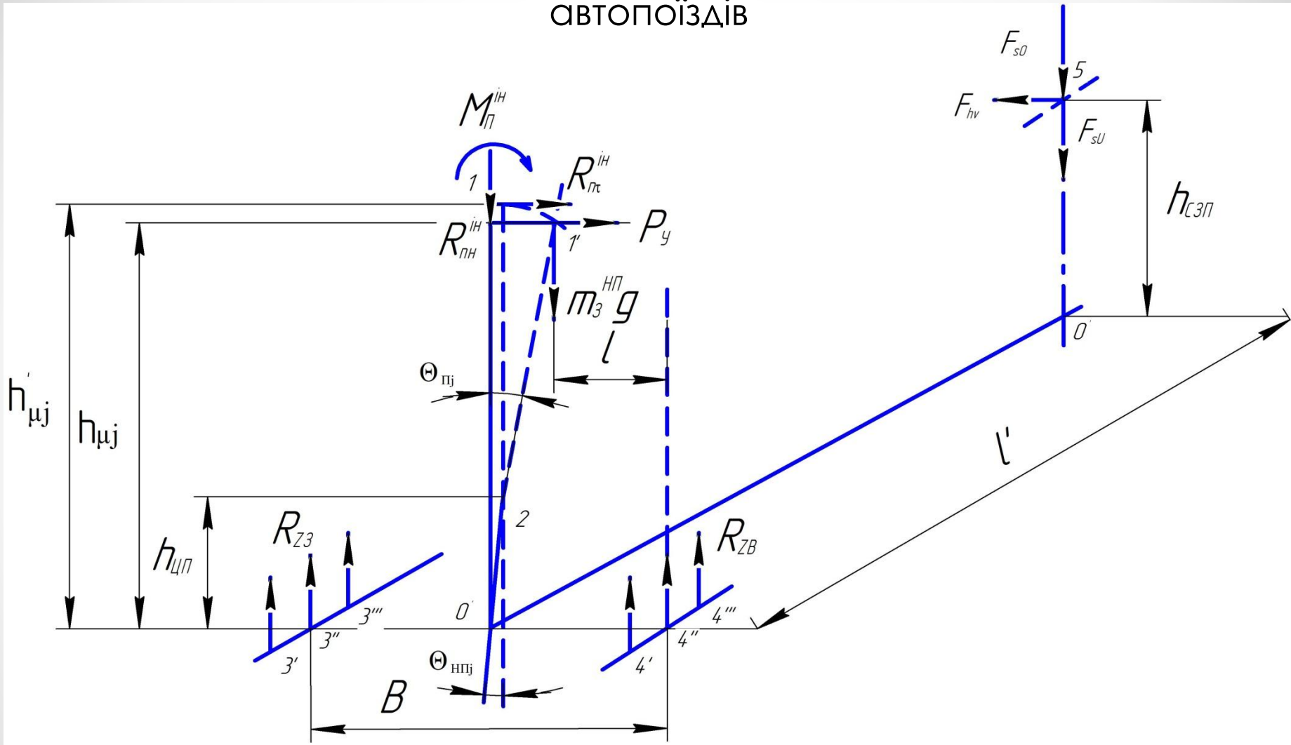
Рис.1. Розрахункова модель Гречанюка М.С. (під редакцією проф. Полякова А.П.)
