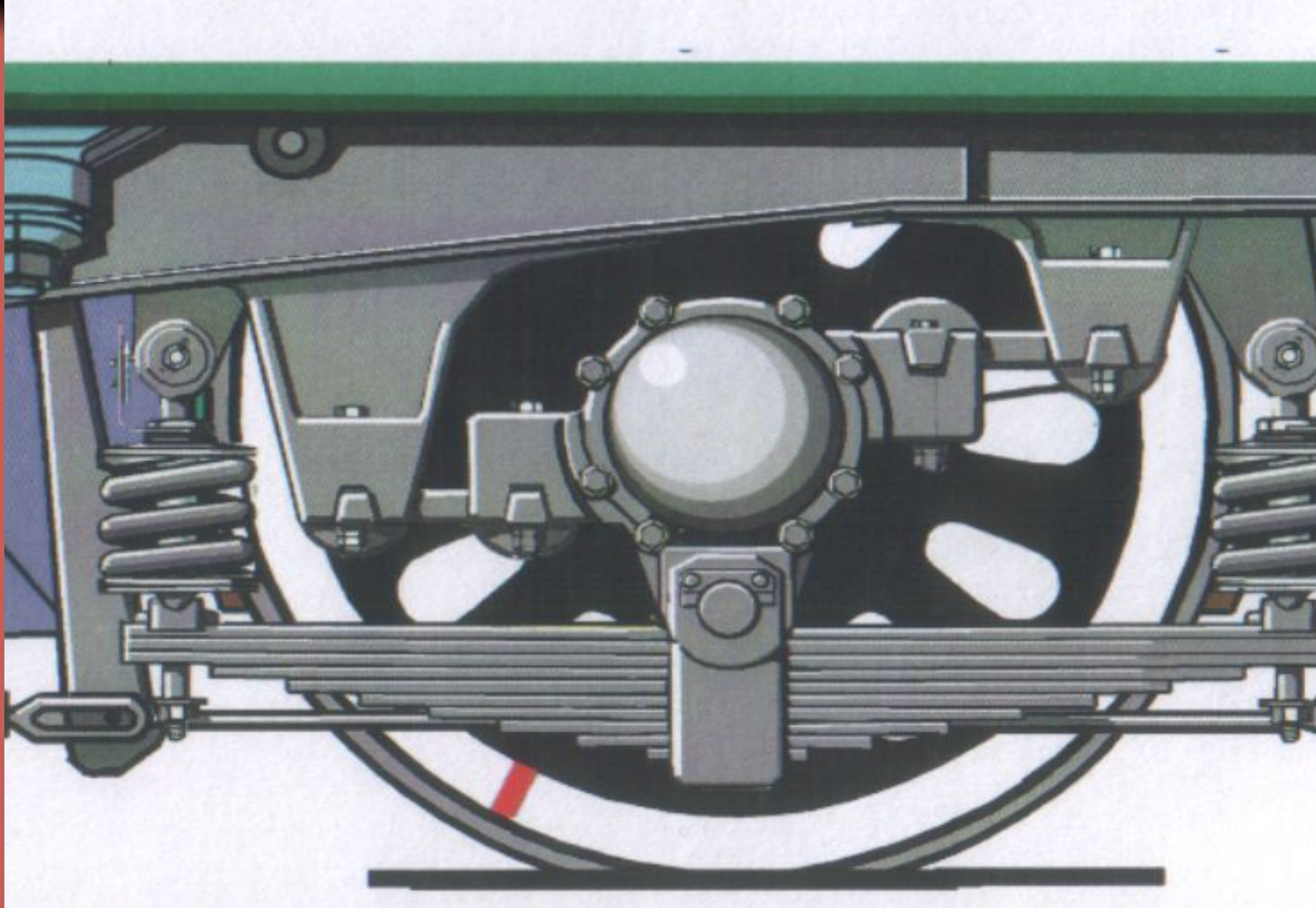
Колесная пара
