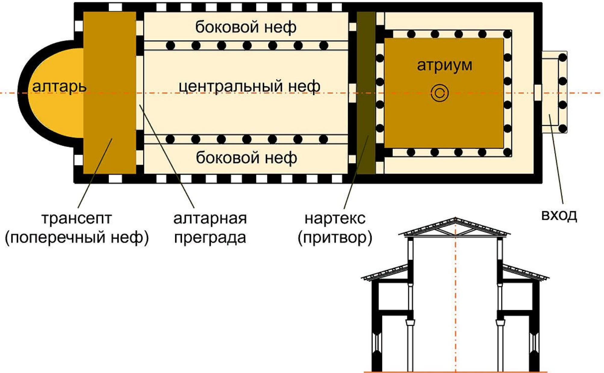
План и конструкция христианской базилики
