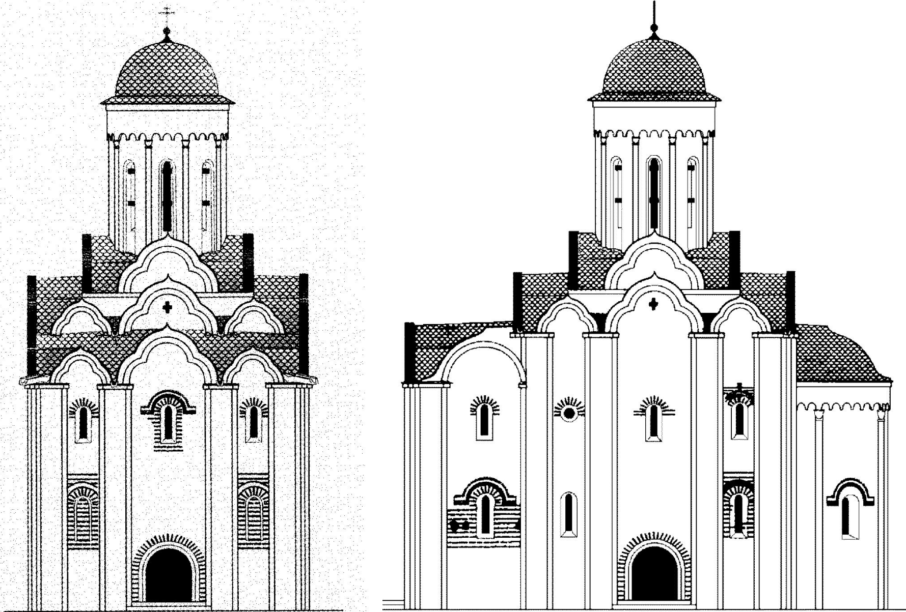
Спасо-Преображенский собор Спасо-Евфросиньева монастыря в Полоцке. Западный и южный фасады. Реконструкция (по В.В. Ракицкому)
