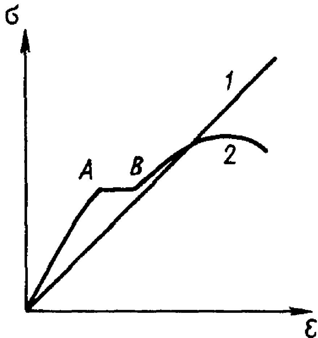
Зависимость деформации от напряжения А 1 — стекло; В 2 - сталь
