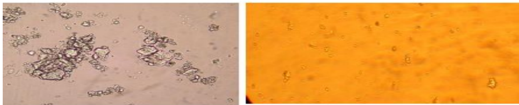
Рис. 2. Комплекс соединений кальция
