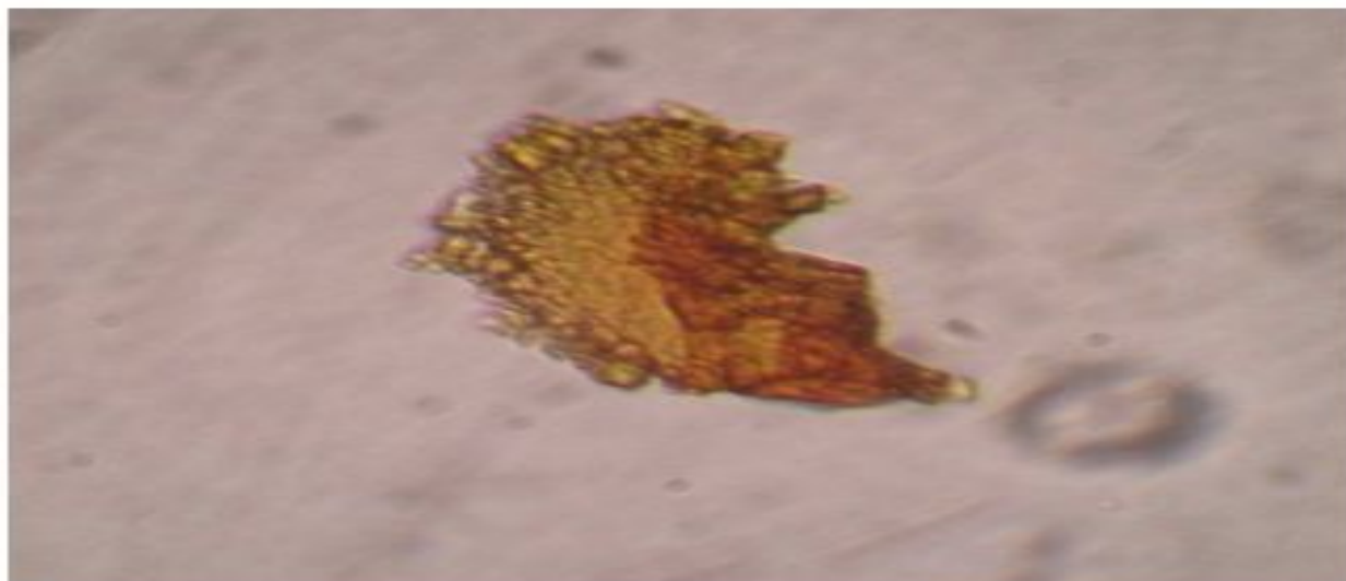
Рис. 1. Одиночный комплекс соединений меди (сульфид меди)
