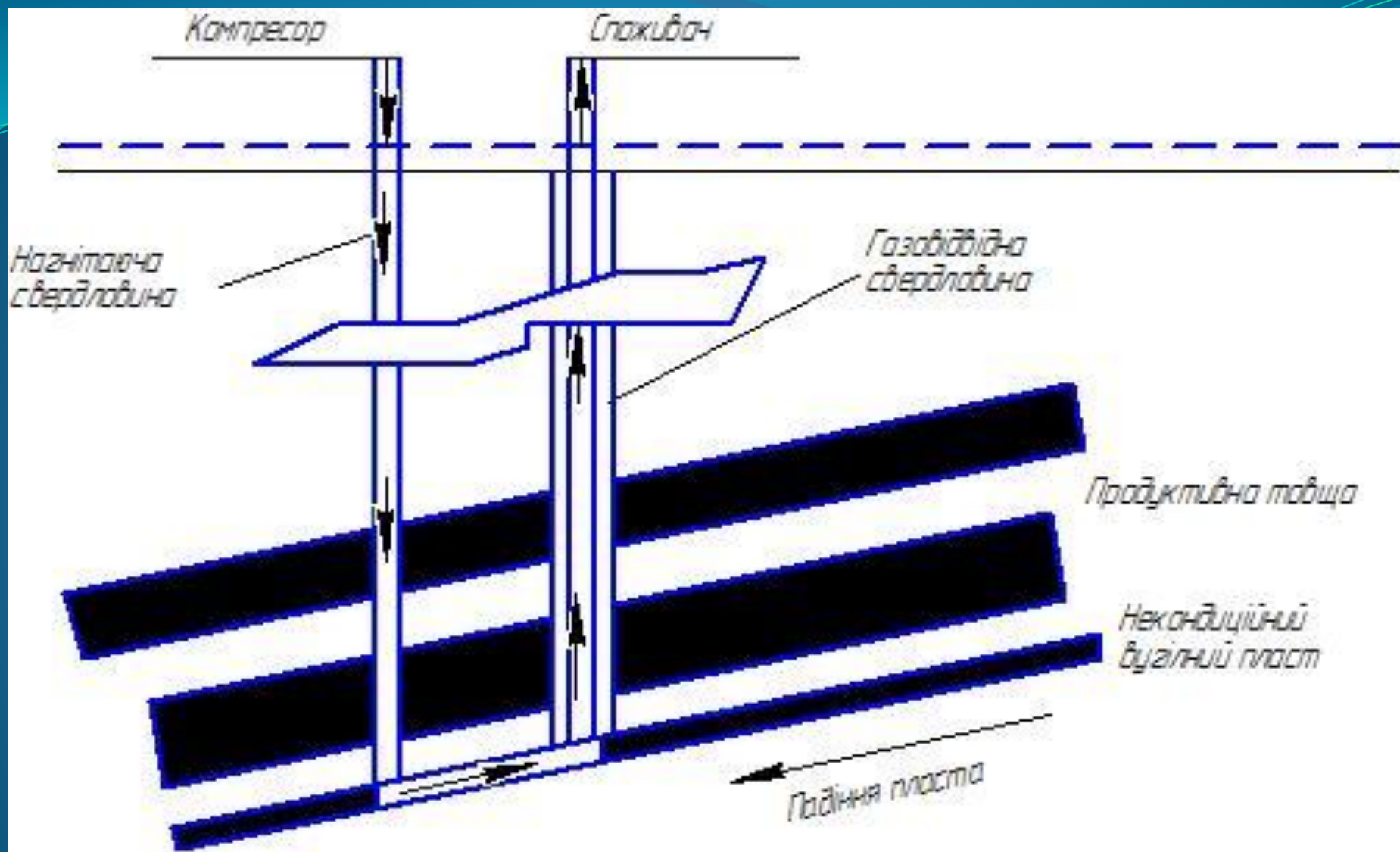
Принципова схема підземної газифікації
