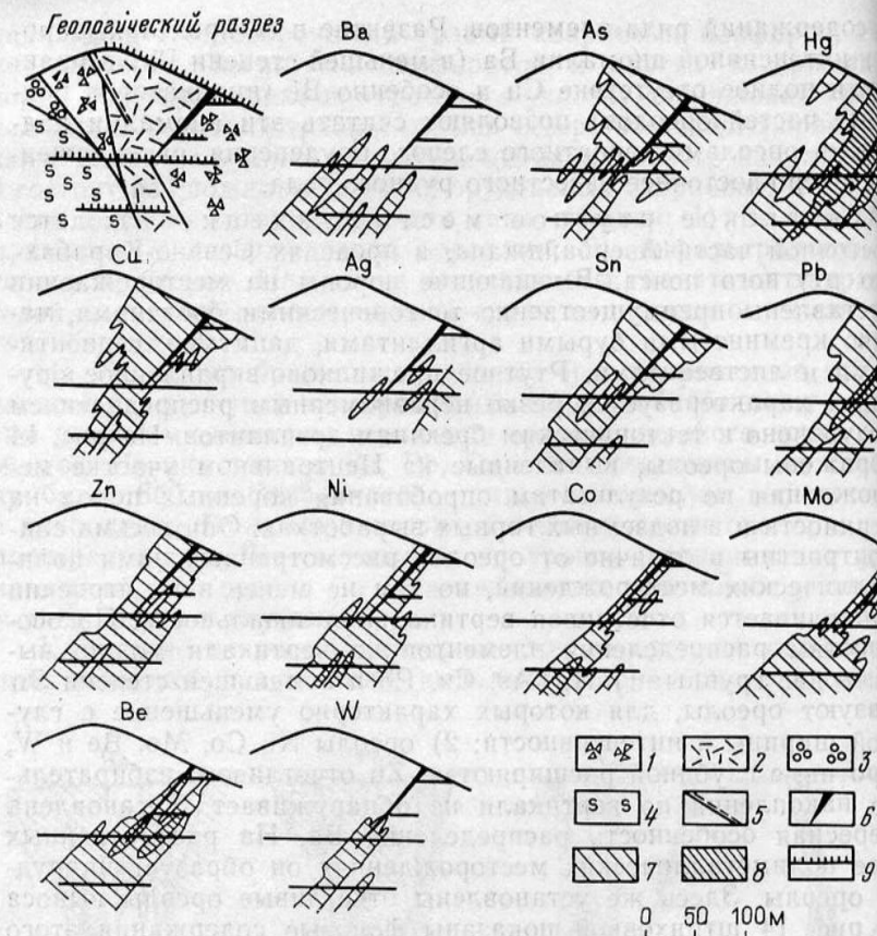
Рис. 14. Первичные ореолы в разрезе:
