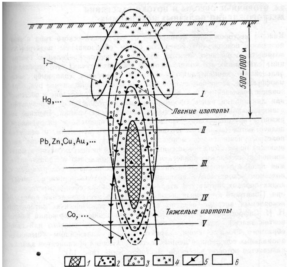
Рис. 12. Обобщенная схема первичного ореола гидротермального месторождения: 1 — рудное тело; 2 — ореол свинца; 3 — ореол ртути; 4 — ореол йода; 5 — ореол кобальта; 6 — современная денудационная поверхность. Римскими цифрами обозначены номера горизонтов
