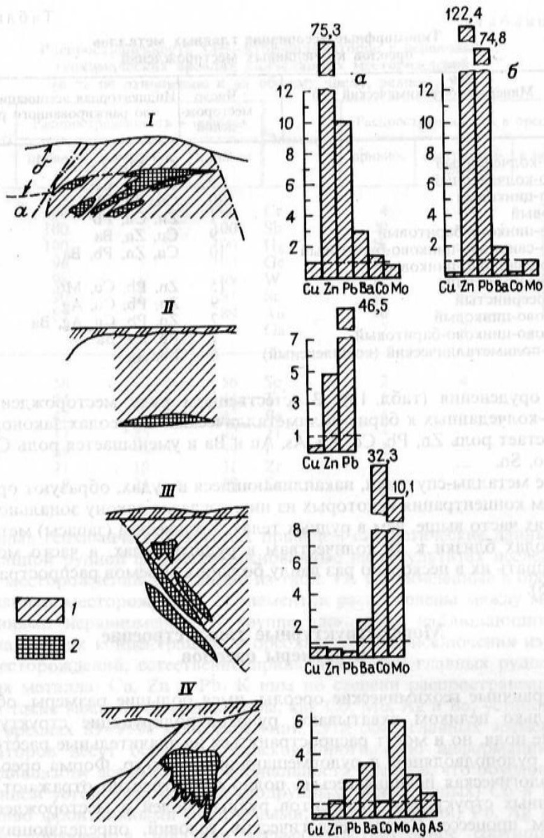
Рис. 5. Соотношение запасов металлов в рудных телах (принятых за единицу) и первичных геохимических ореолах Маднелевского (I), Лениногорского, Быструшинская залежь (II), Гайского (III) и Озерного (IV) месторождений: 1 – площадь ореола, в пределах которой подсчитывались запасы; 2 – рудное тело; зоны: а – подрудная, б – надрудная
