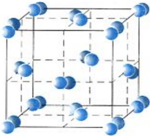
Молекулярная кристаллическая решётка йода
