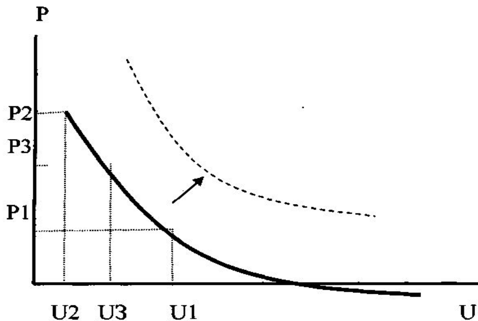
рис. 1. Кривая Филлипса.
