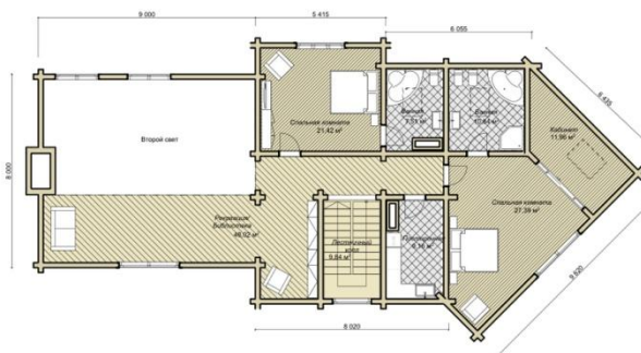
2 этаж
