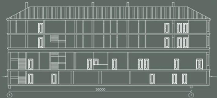
Разрез 1-7
