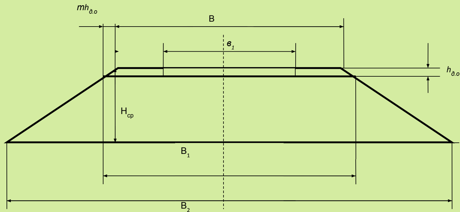
Расчетная схема № 2
