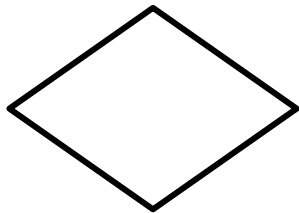
Ветвление, выбор
