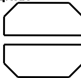
Граница цикла
