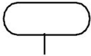
Начало программы
