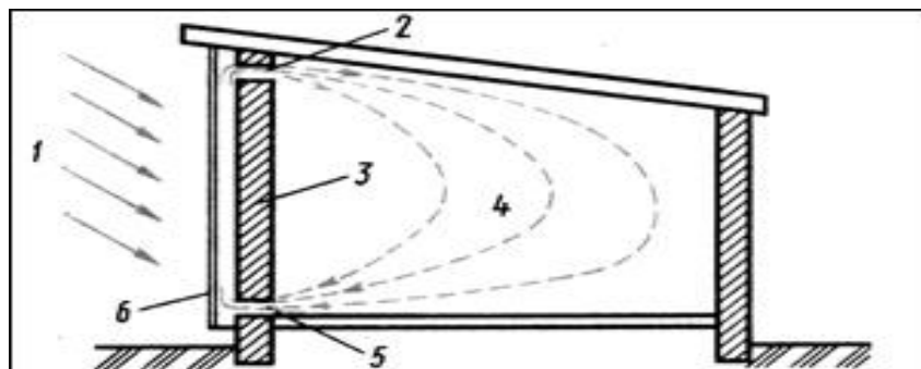
Рис. 5.1. Схема пассивного использования энергии солнца (конструкции Тромба-Мишеля): 1 — солнечная радиация; 2 — поток теплого воздуха в жилое помещение; 3 — наружная стена; 4 — жилое помещение; 5 — поток охлажденного воздуха из жилого помещения; 6 — стеклянная панель
