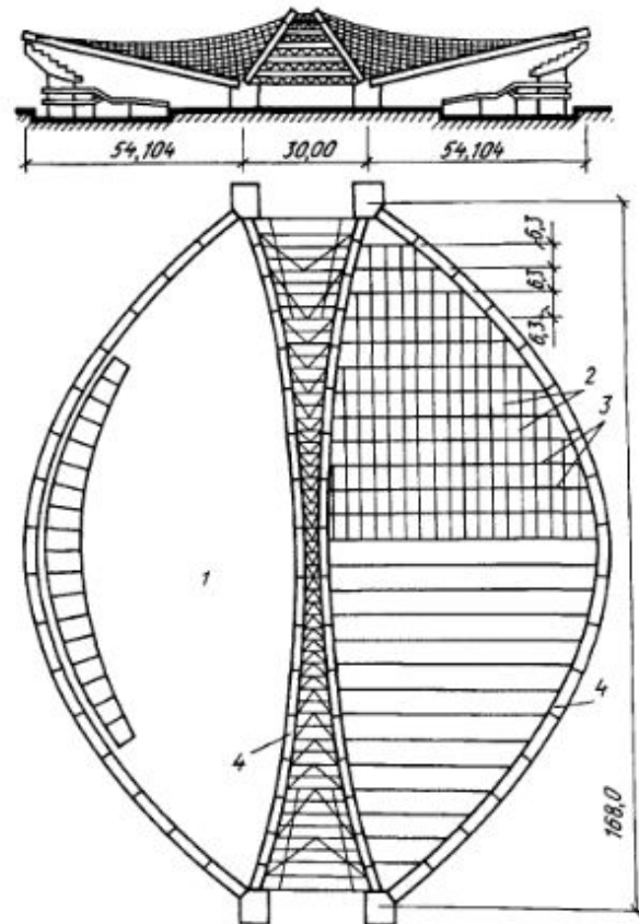
Покрытие седловидными мембранами изотрелка в Москве 1 — металлическая мембрана; 2, 3 — элементы постели; 4 — металлические арки
