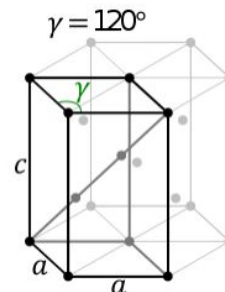
Дважды-объёмноцентрированная (Ромбоэдрическая)
