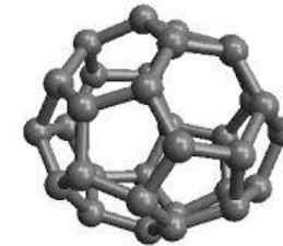
Фуллерен C32
