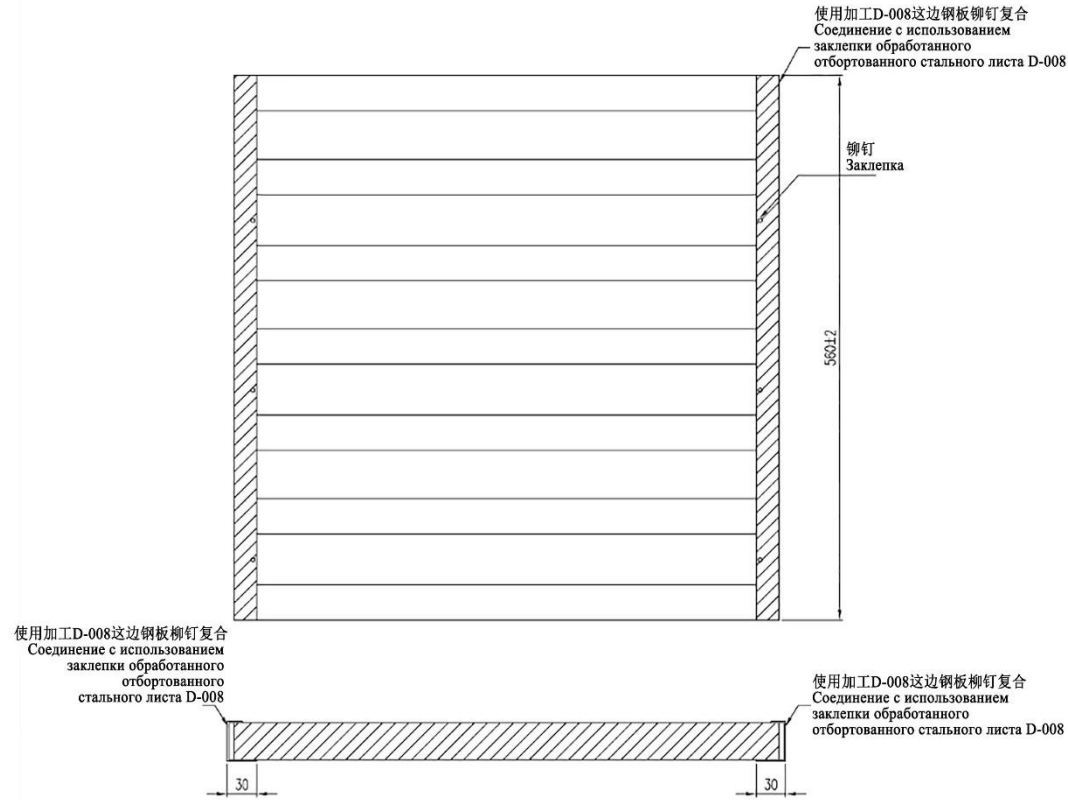
组装示意图 Схема сборки
