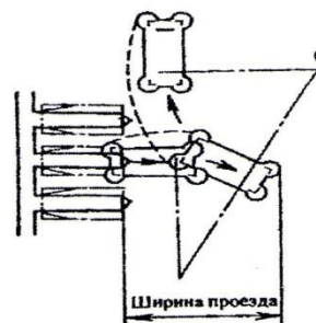
Установка автомобиля на тупиковые посты зон ТО и ТР, оборудованные смотровыми канавами
