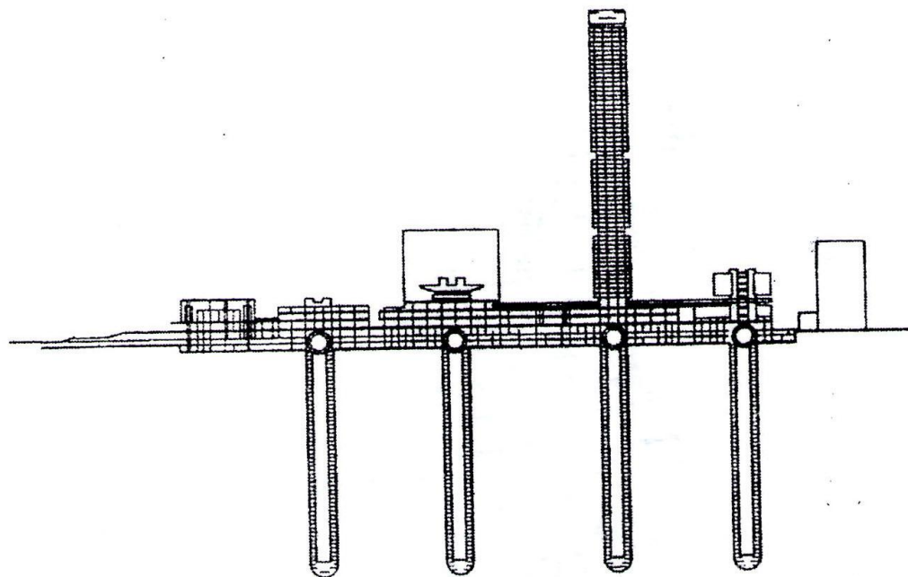
Наземно-подземные механизированные гаражи-шахты. Проектное предложение для Нью-Йорка
