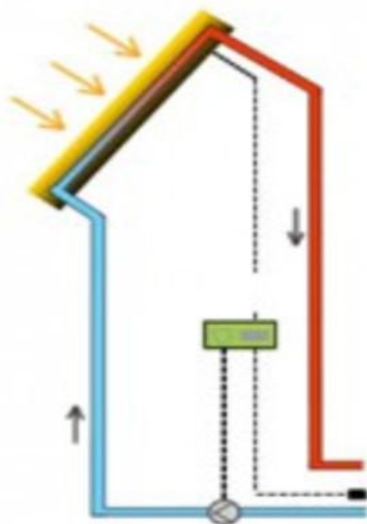
Солнечно-водяной коллектор
