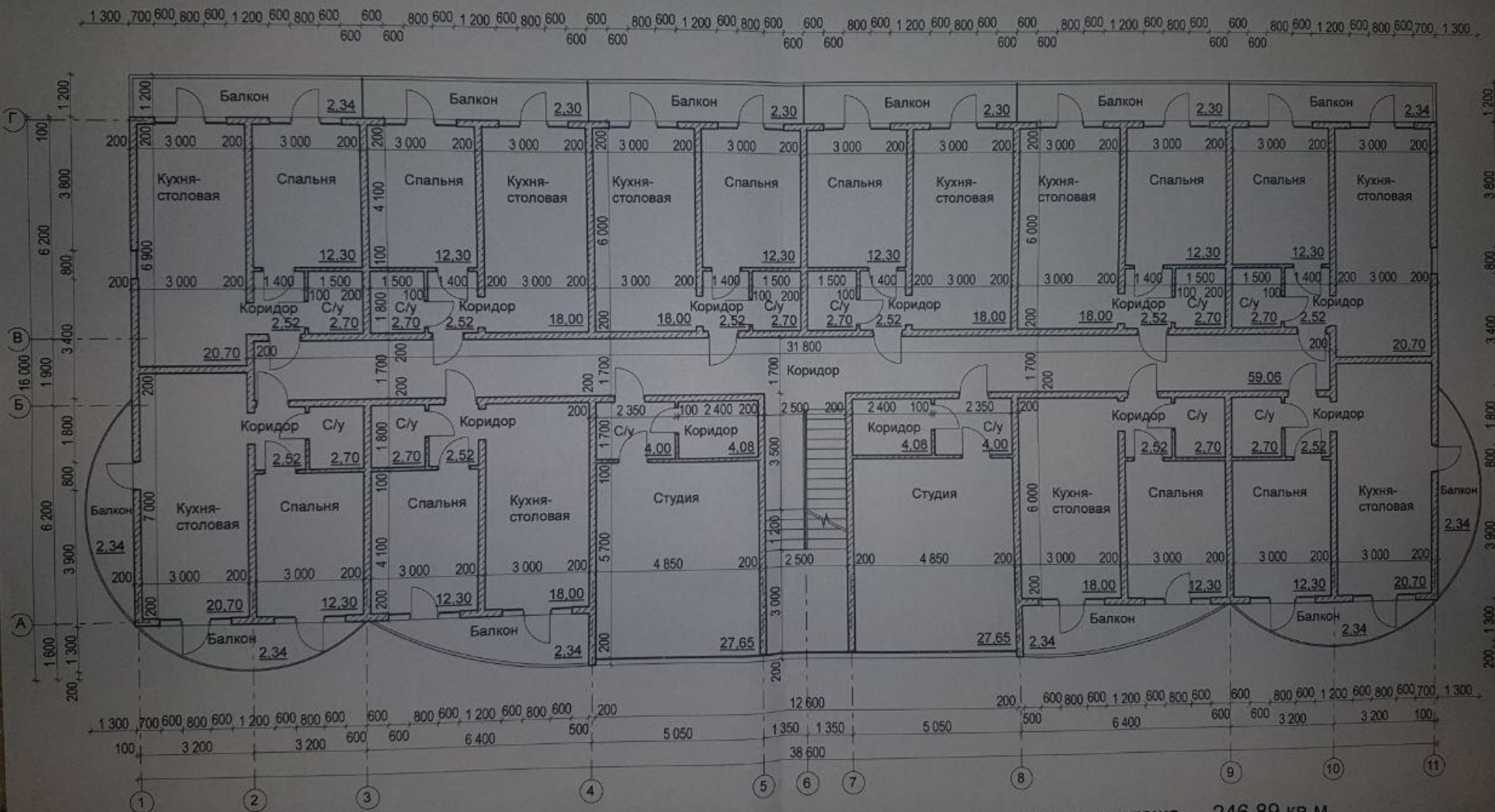
ПЛАН ВТОРОГО, ТРЕТЬЕГО ЭТАЖА
