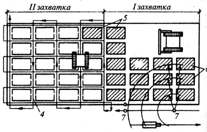
Извлечение блоков краном
