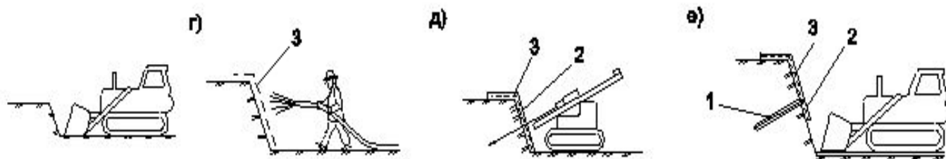
Рис. Технологическая последовательность нагельного способа горизонтального армирования стенки из торкретбетона:
