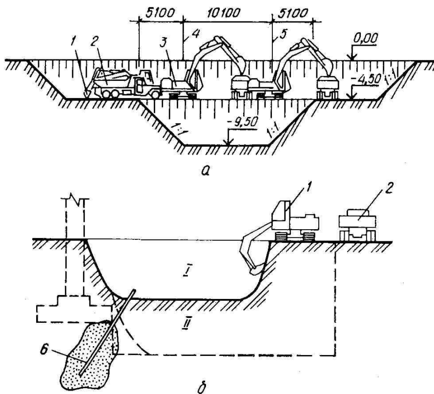
Рис. Разработка грунта в котловане в два яруса:
