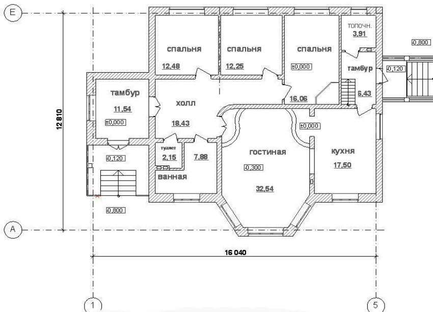
План на отметке 0.000 М 1:100
