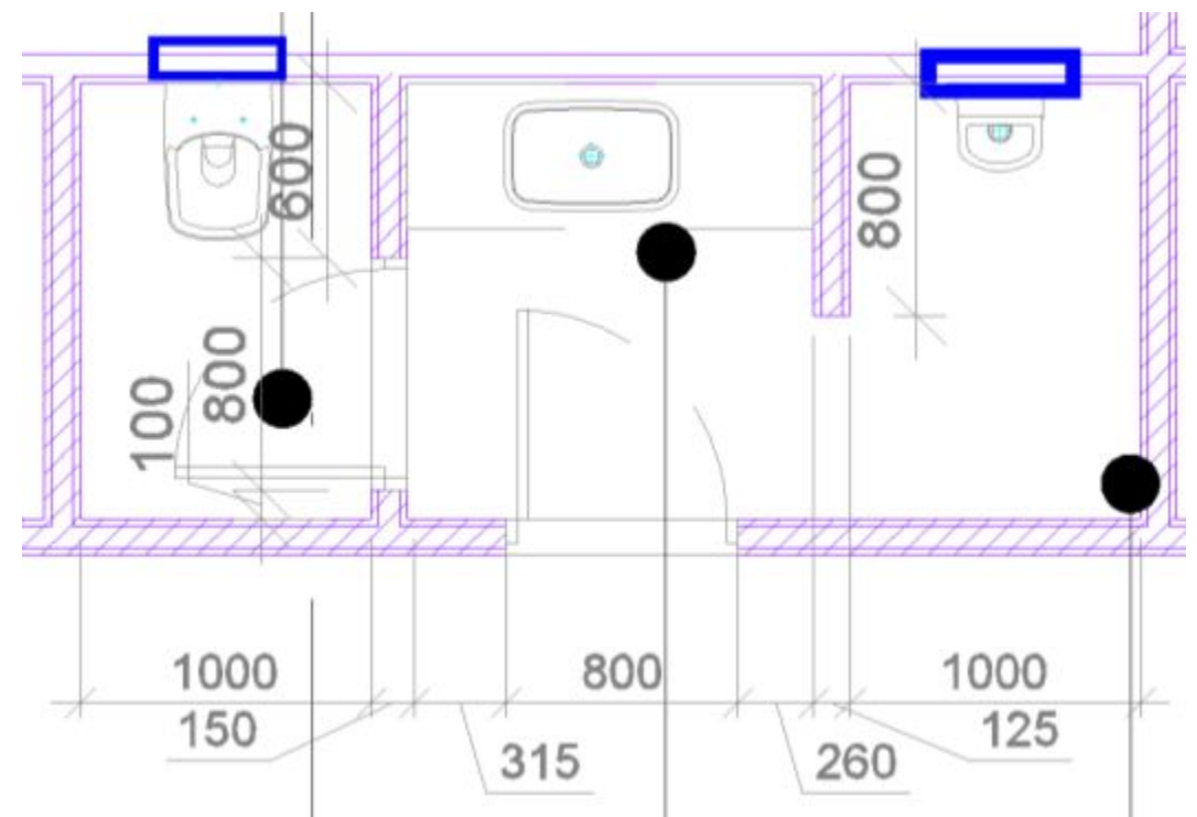
План помещений с размерами
