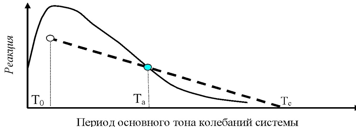
Рис.5. Соотношение спектров воздействия (сплошная кривая) и состояний системы (пунктир)
