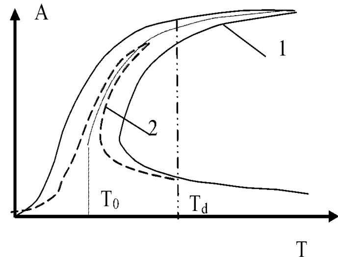
Рис.4. АЧХ нелинейного осциллятора для малого(1) и большого(2) демпфирования
