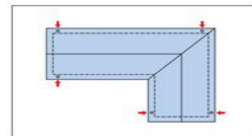
L-образная кровля
