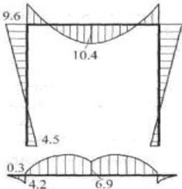
Эпюра моментов при раздельном расчете рамы и фундаментной балки
