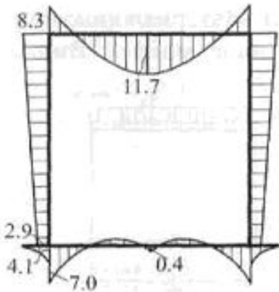
Эпюра моментов при последовательном возведении конструкции
