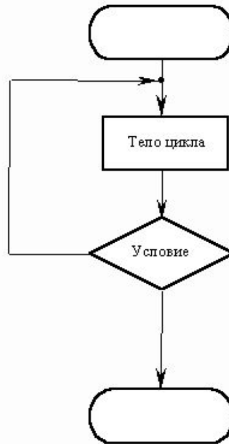
Цикл с послеусловием
