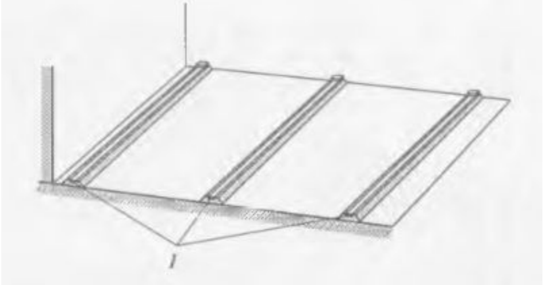
Рис. 11. Укладка маяков на полу: 1 — деревянные рейки
