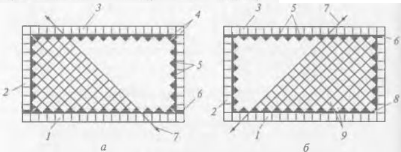
Рис. 8. Диагональная облицовка плитками; а — вставки треугольные; б — четвертушки в углах; 1 — нижний ряд фриза; 2, 3 — соответственно вертикальная и верхняя ленты; 4, 5 — треугольные плитки соответственно в углах и по периметру фриза; 6 — вставка из неполномерных плиток; 7 — причальный шнур; 8 — четвертушки в углах фриза; 9 — зеркало уложенной плитки
