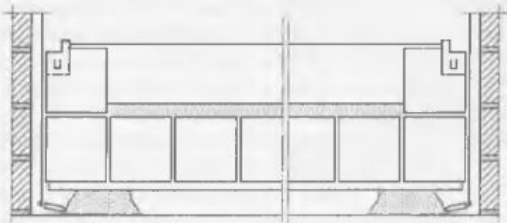
Рис. 7. Облицовка маячного ряда
