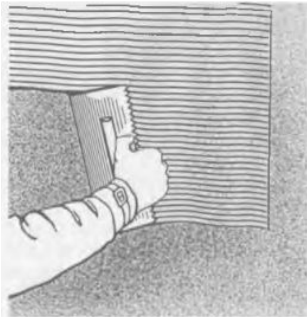
Рис.9. Нанесение клея на поверхность стены зубчатой гладилкой
