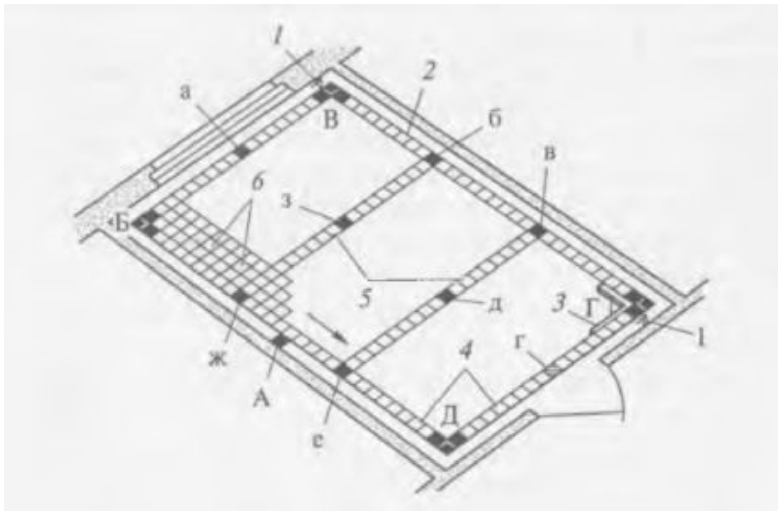
Рис. 18. Размещение маяков и направление захваток: а — реперный маяк; б...д — угловые фризозые маяки; а...з — промежуточные маяки; 1 — стальной штырь; 2 — причальный шнур; 3 — угольник; 4 — фризозый ряд; 5 — маячные полосы-провесы; 6 — полоса-захватка
