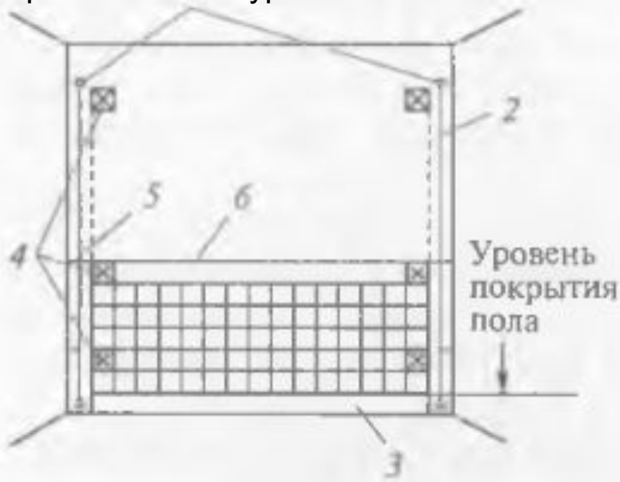
Рис. 6. Облицовка стен: 1— стальные штыри; 2— шнур; 3— рейка; 4— маячные плитки; 5 — штырь, для крепления причалки; 6 — причальный шнур
