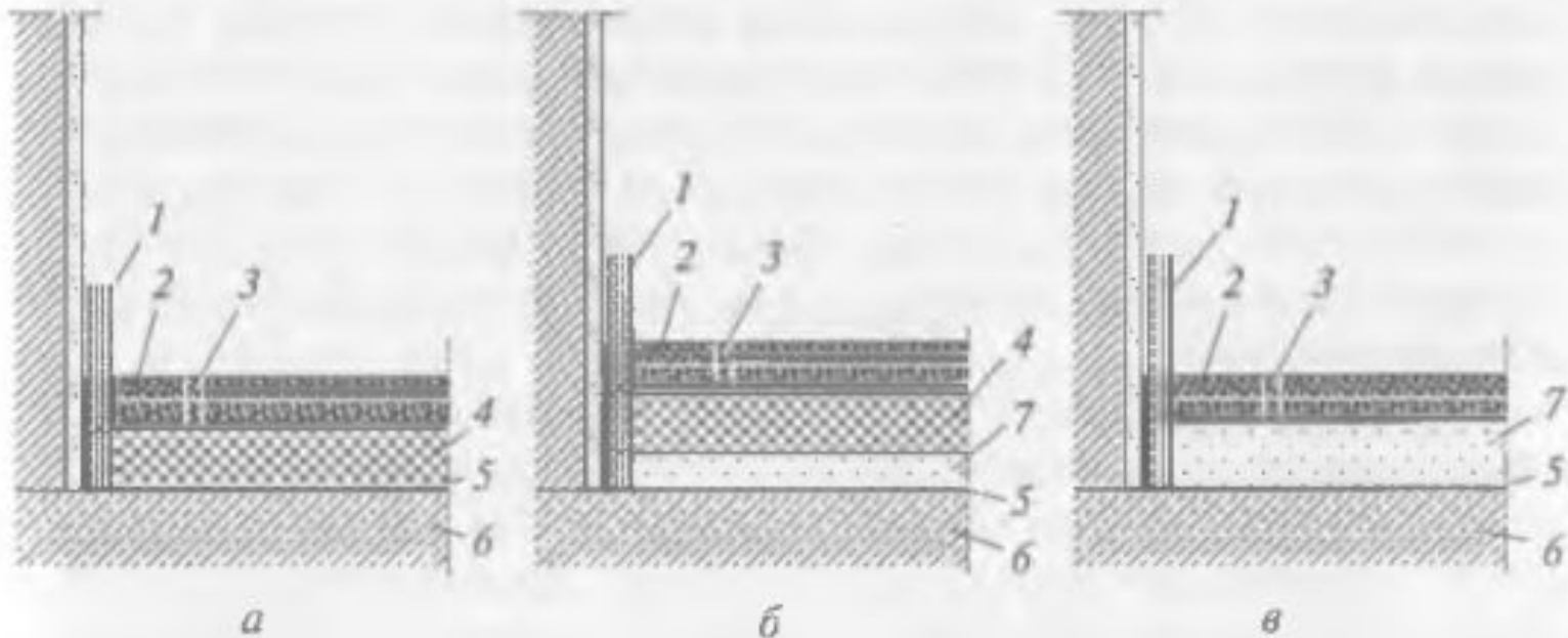
Рис. 16. Системы сборных полов: а — пол сборный на изолирующем слое; б — пол сборный на изолирующем слое с выравнивающей засыпкой; в — пол сборный на выравнивающем слое; 1 — лента кромочная из минеральной ваты; 2 — панели гипсокартонные; 3 — зажим;
