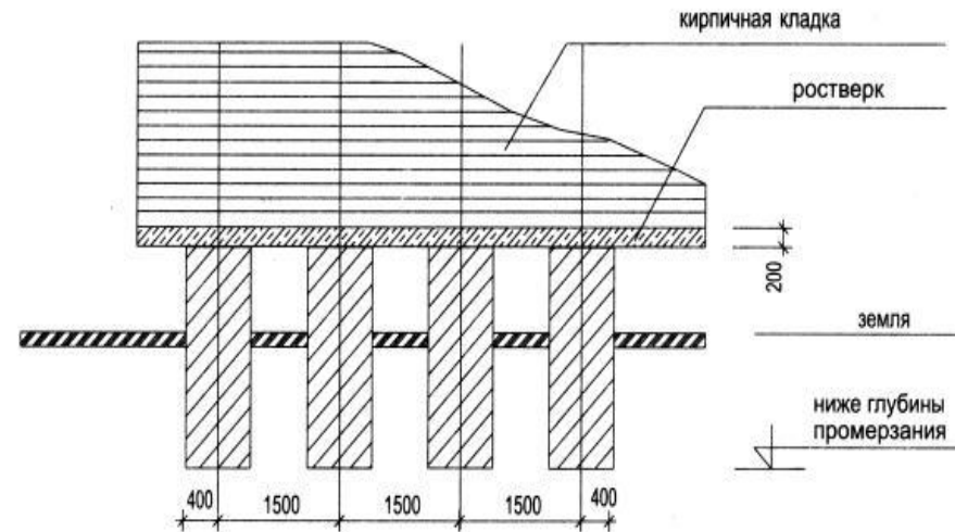
Столбчатые фундаменты
