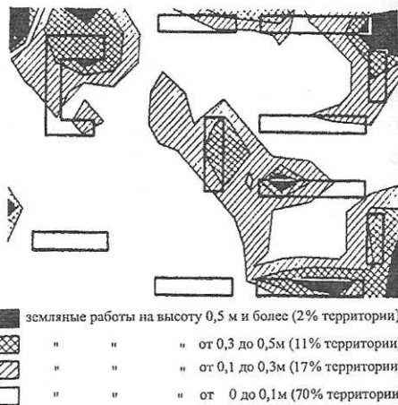
Рис. Картограммы земляных работ, выполненные по разным вариантам вертикальной планировки
