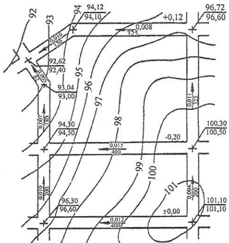
Рис. Фрагмент схемы вертикальной планировки
