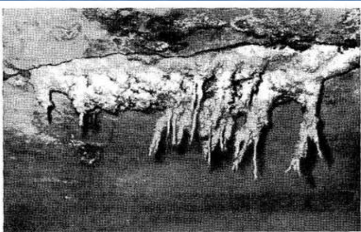
Рис. 1.3. Свисающие с перекрытия сталактиты — результат углекислой коррозии
