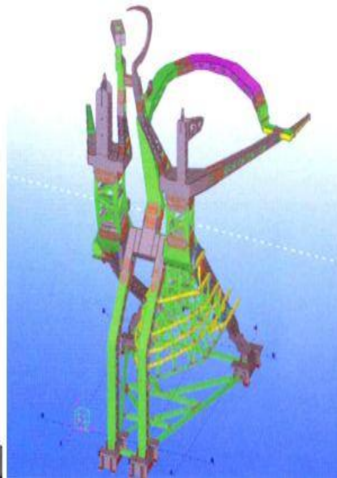
Скульптура «Рабочий и колхозница»: слева – фрагменты каркаса, справа – модель в программе Tekla Structures
