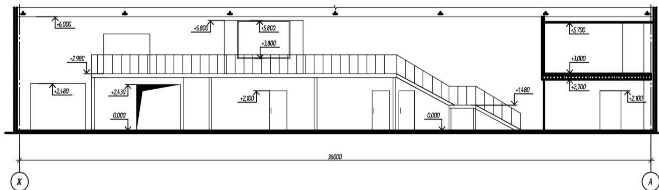
Разрез 3-3
