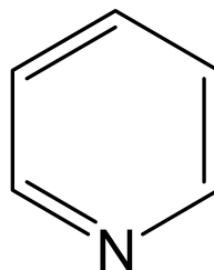
пиридин
