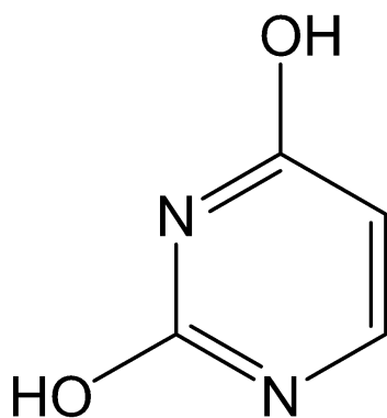
урацил (2,4-диоксипиримидин)
