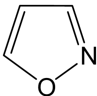
изоксазол
