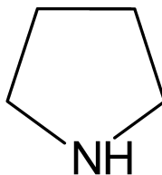
пирролидин
