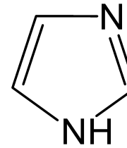
имидазол
