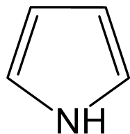
пиррол
