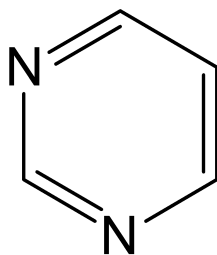
пиримидин
