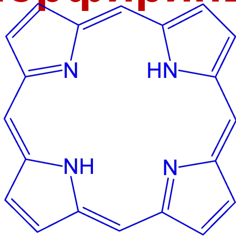
Порфин
