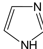
имидазол
