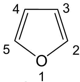
фуран
