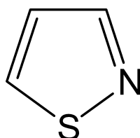
изотиазол
