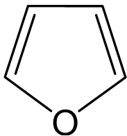
фуран
