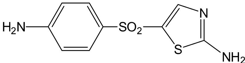
Промизол
