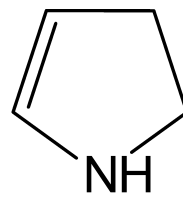
2,3- и 2,5-дигидропиррол (пирролин)
