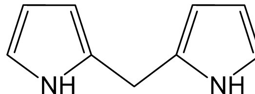
дипиррилметан
