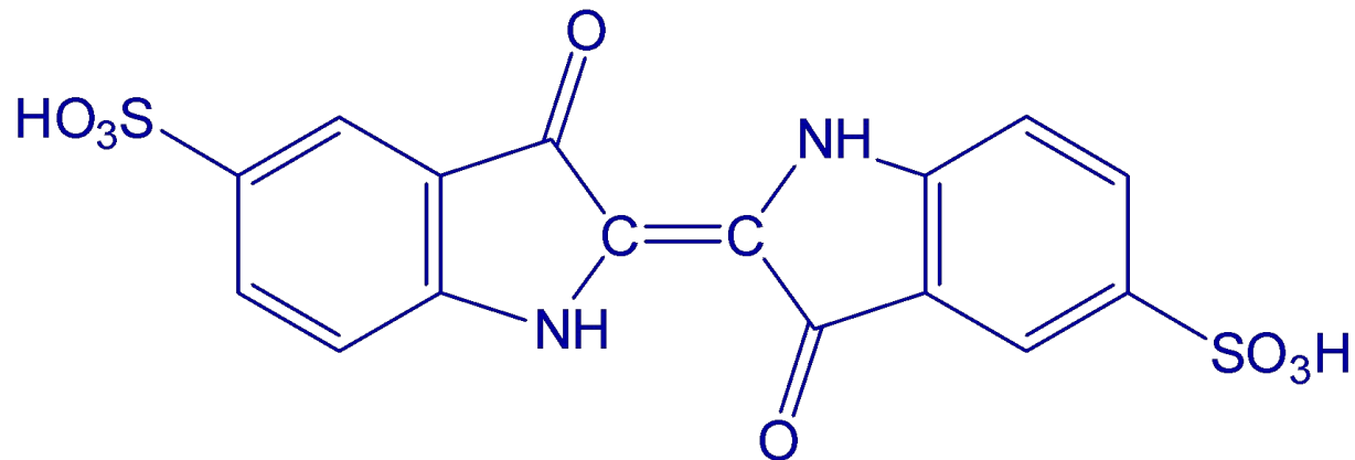
5,5'-индигосульфокислота
