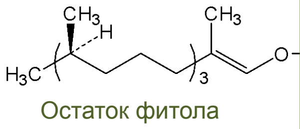
Хлорофилл а
