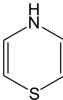
тиазин
