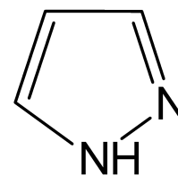
пиразол
