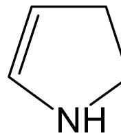
пирролин
