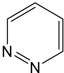
пиридазин
