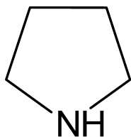
пирролидин
