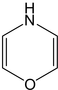
оксазин
