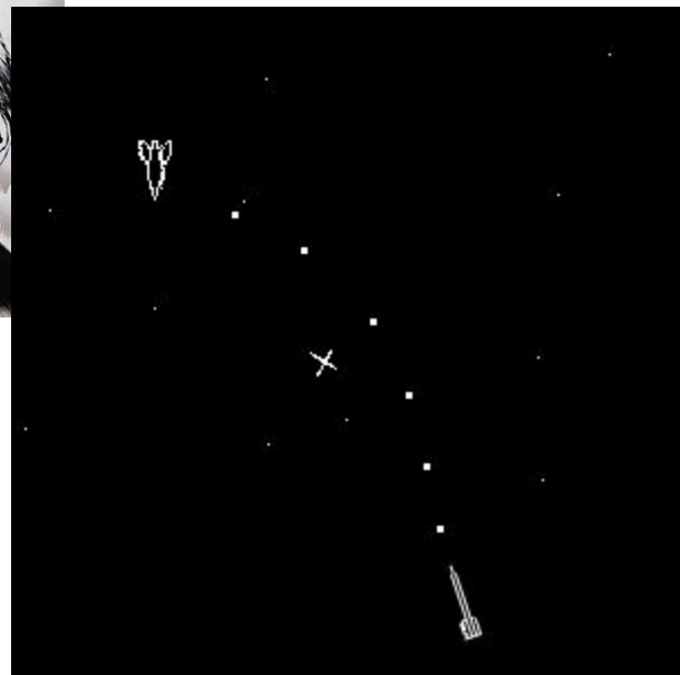
Spacewar!
