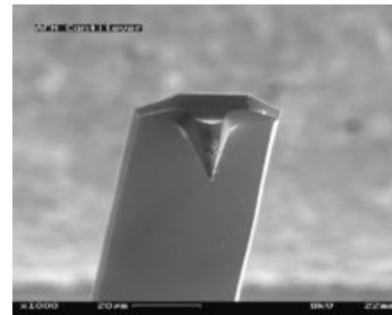
Кантилевер атомно-силового микроскопа
