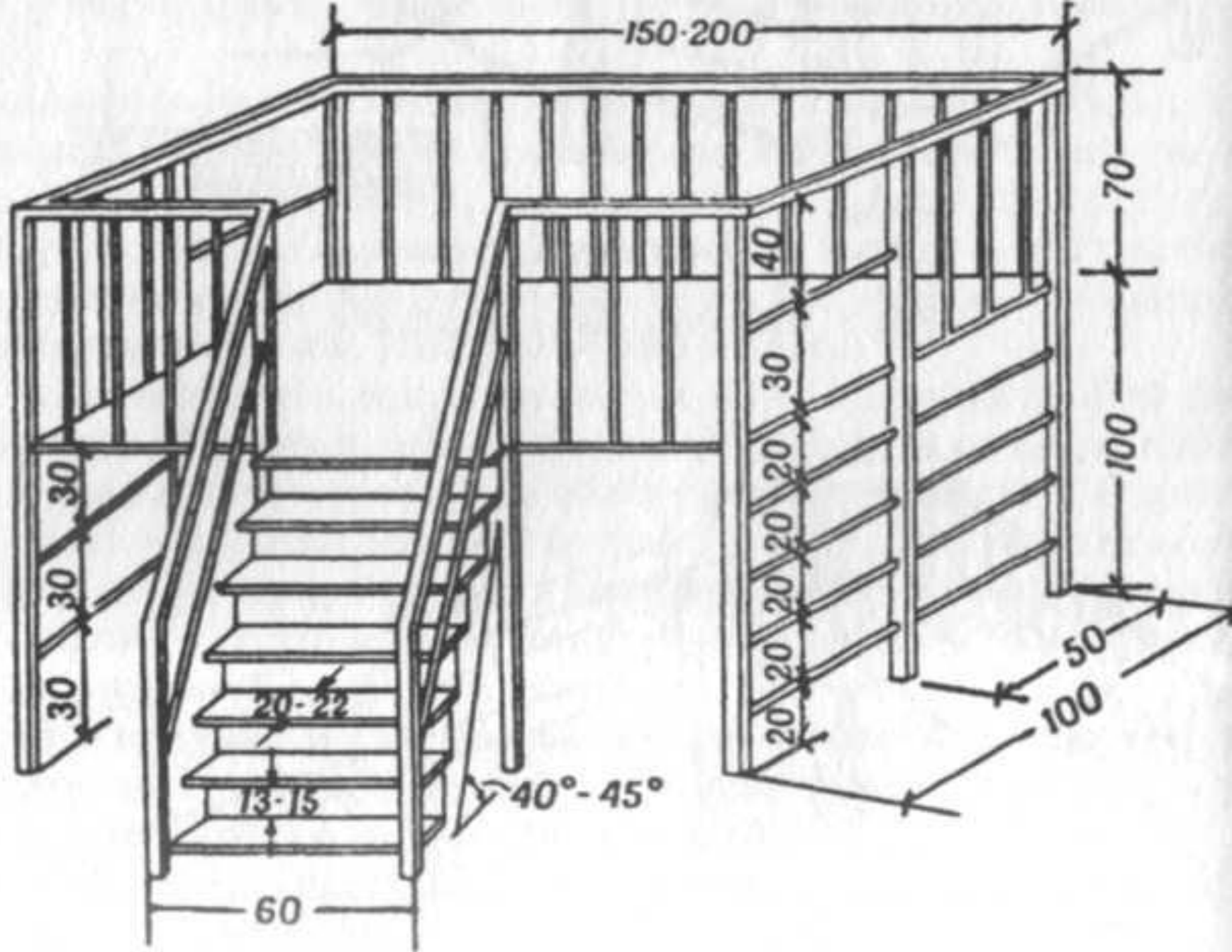
Рис. 7. Вышка для лазания детей младшего возраста
