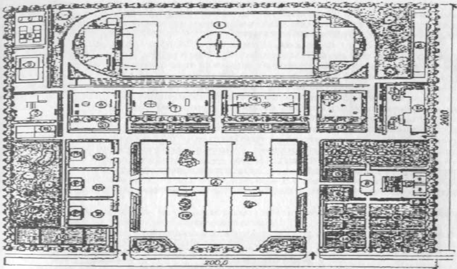
Рис. 11. Схема плана земельного участка (типовой проект) для школы и школы-интерната на 25 классов:
