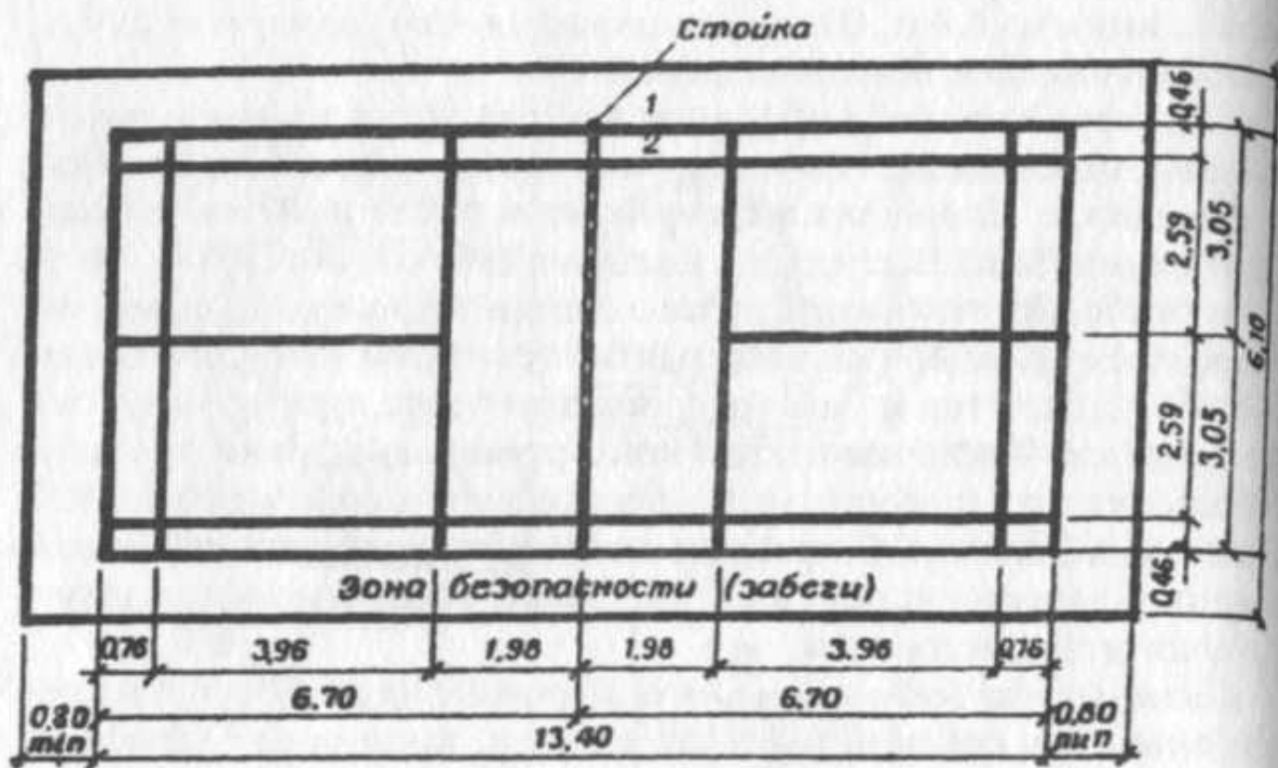
Рис. 16. Площадка для бадминтона (план):
