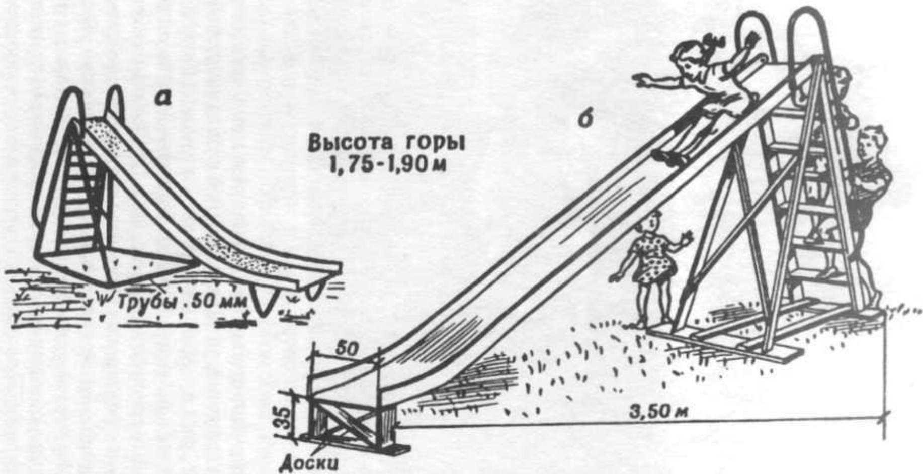
Рис. 34. Детские летние горки: а — из металлических труб; б — деревянные детали
