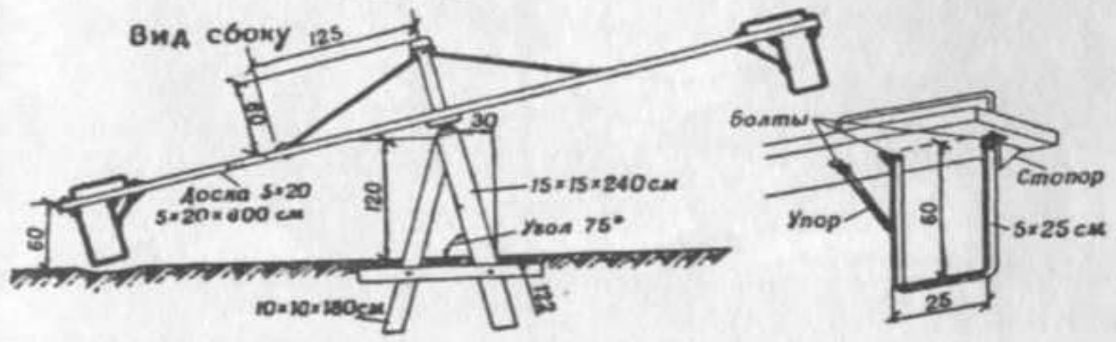
Рис. 31. Наклонная карусель с подножками. Общий вид и детали
