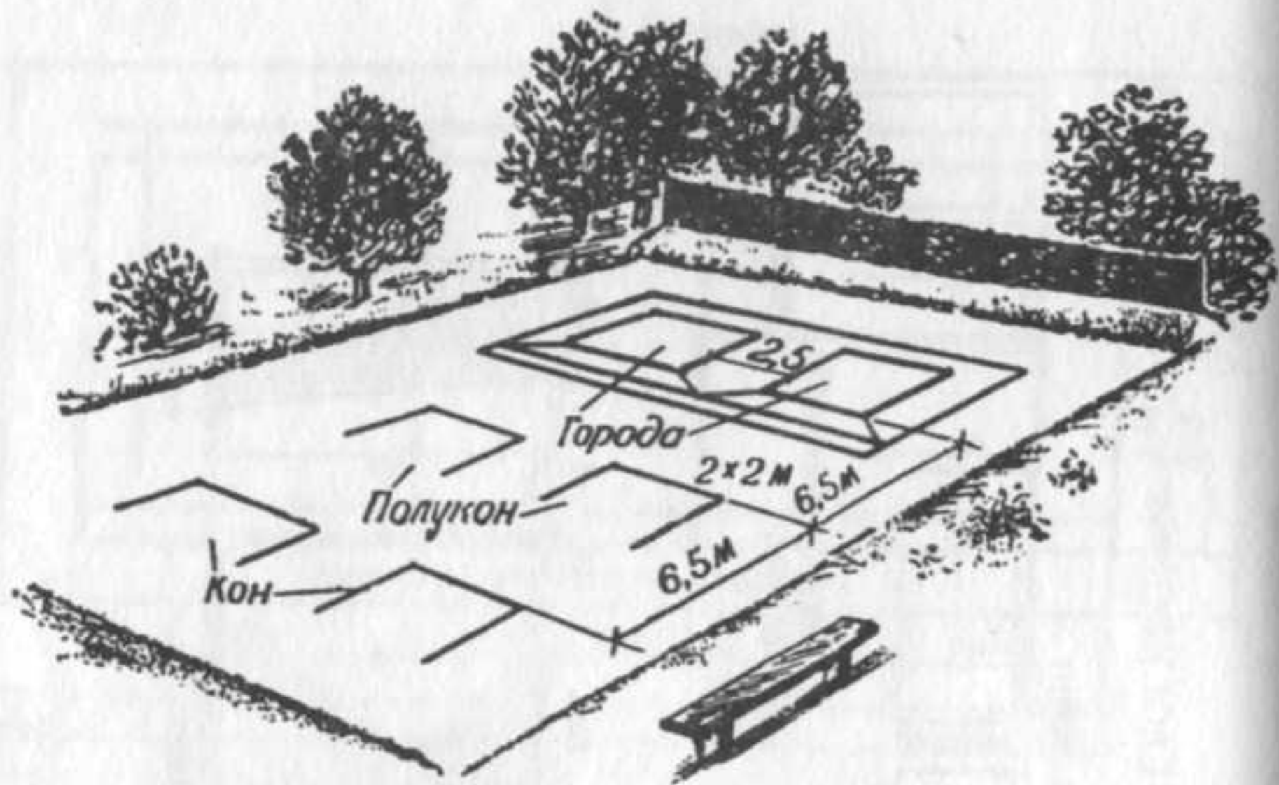
Рис. 18. Площадка для городков (общий вид)
