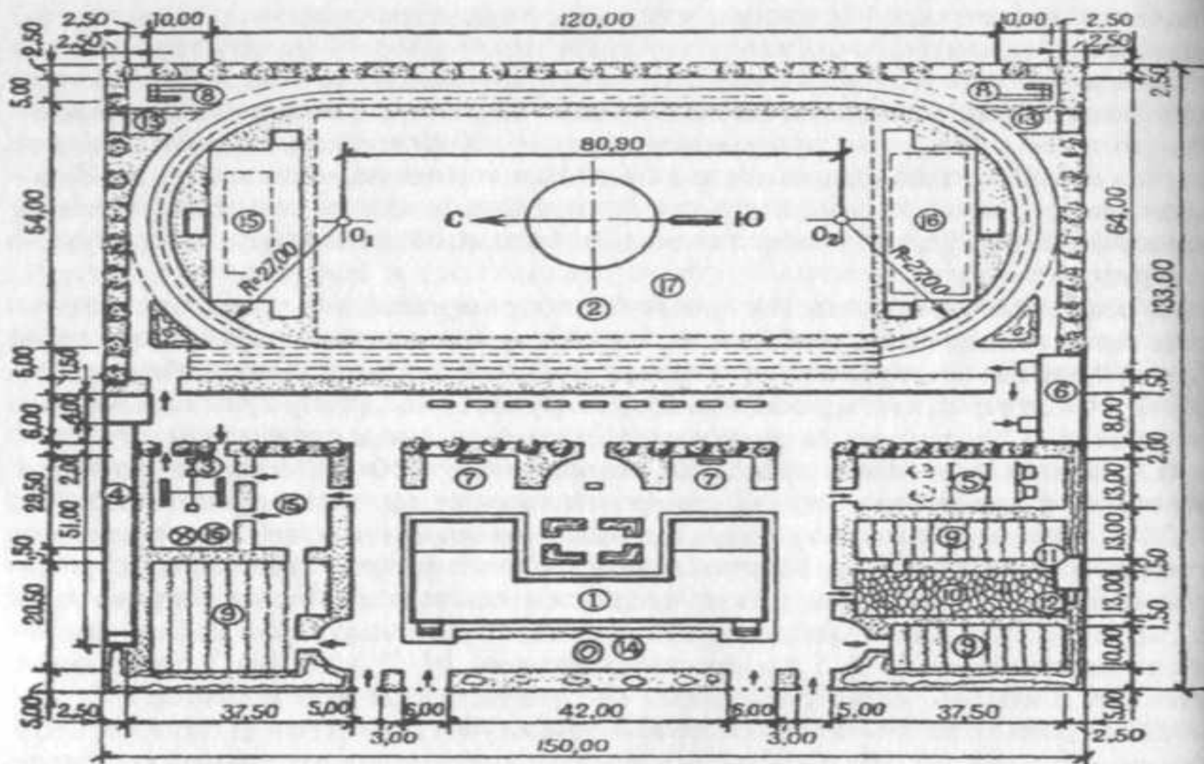
Рис. 10. Схема плана школьного земельного участка площадью 2 га: 1 — здание школы; 2 — спортядро № 1; 3 — гимнастический городок; 4 — тир; 5 — городки; 6 — лыжехранилище; 7 — площадки для младших школьников; 8 — ледяные горы; 9 — огород и сад; 10 — хоз. двор; 11 — сарай; 12 — мусорный ящик; 13 — уборные; 14 — цветы; 15 — площадка для баскетбола; 16 — площадка для волейбола; 17 — поле для футбола 90x50 м
