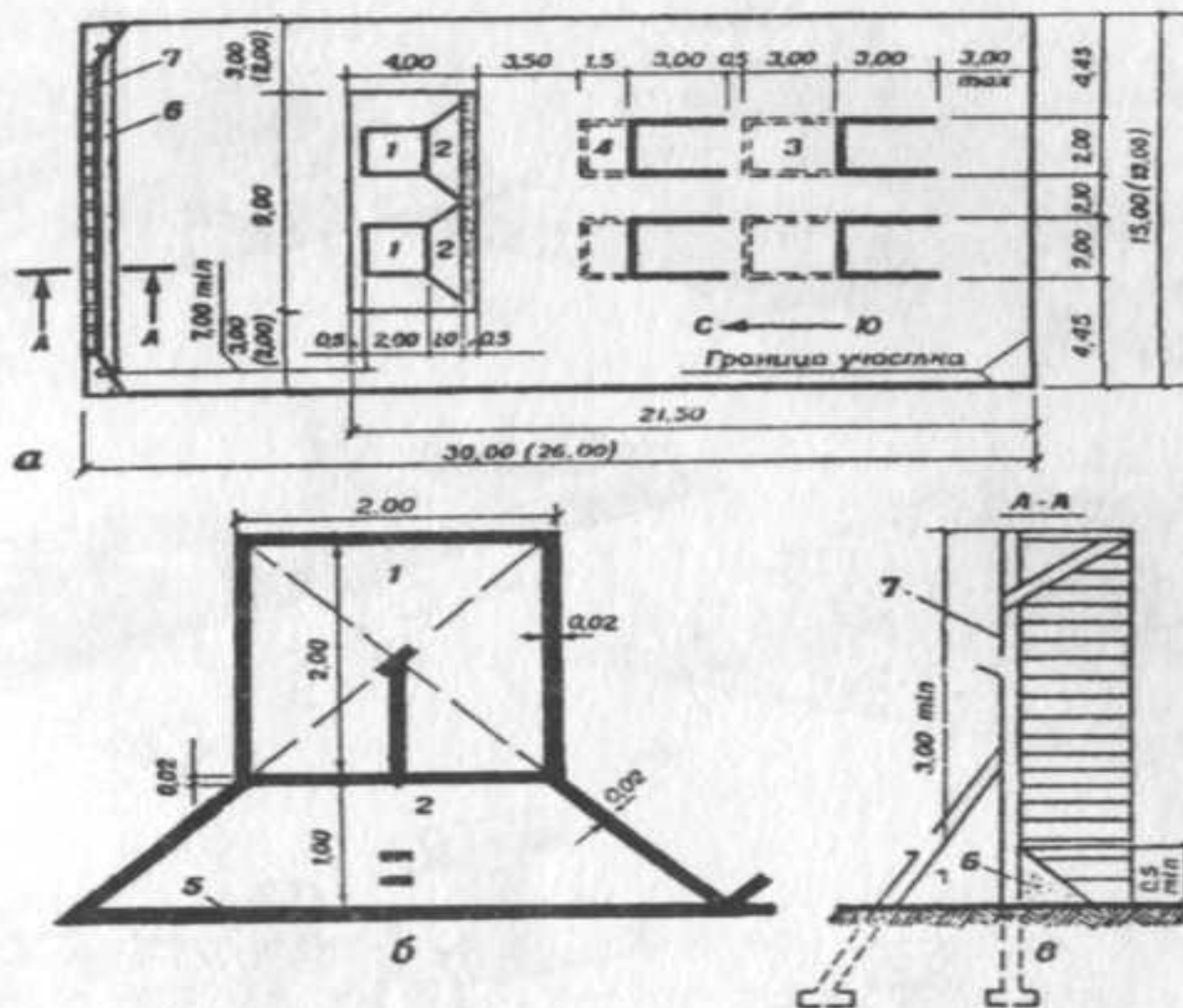
Рис. 19. Площадка для городков:
