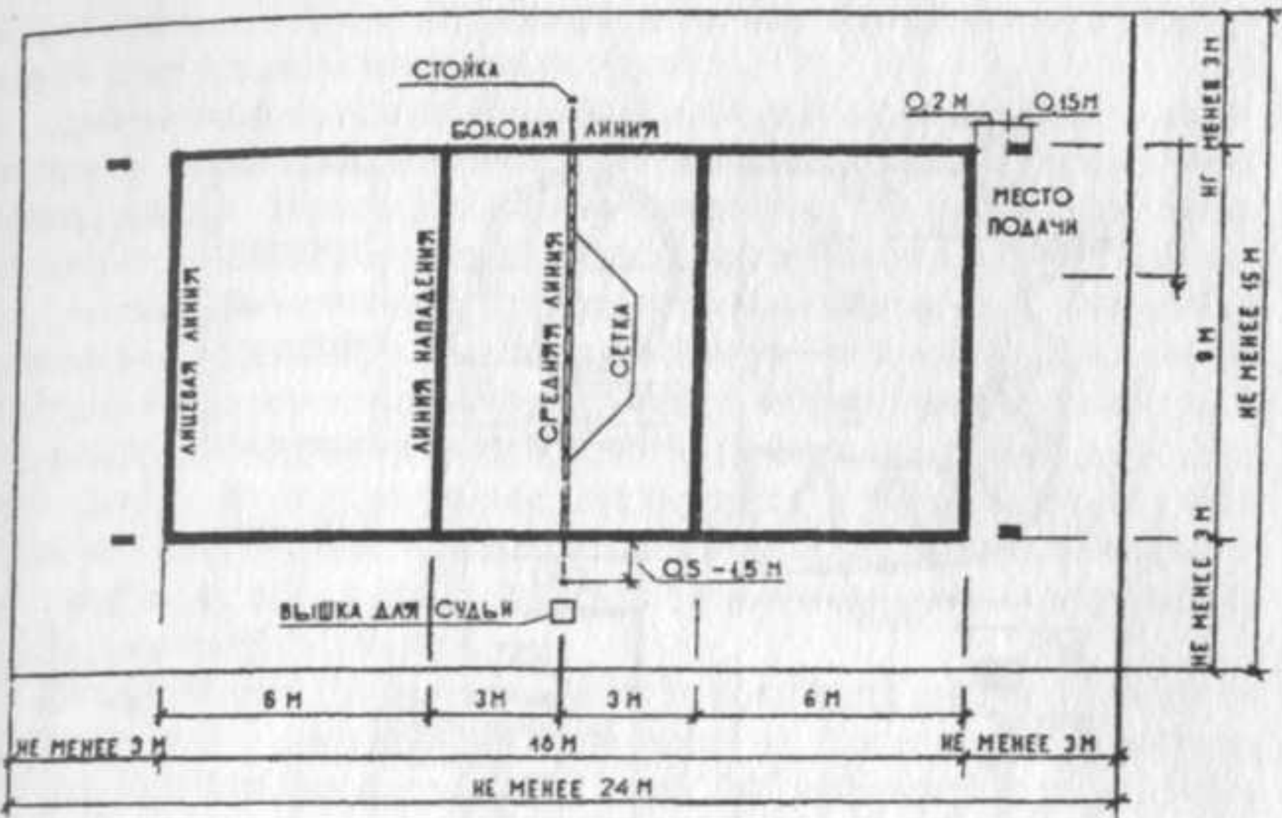
Рис. 13. Волейбольная площадка (план, размеры)
