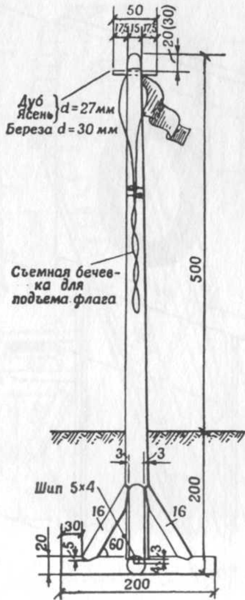
Рис. 27. Столб для лазания
