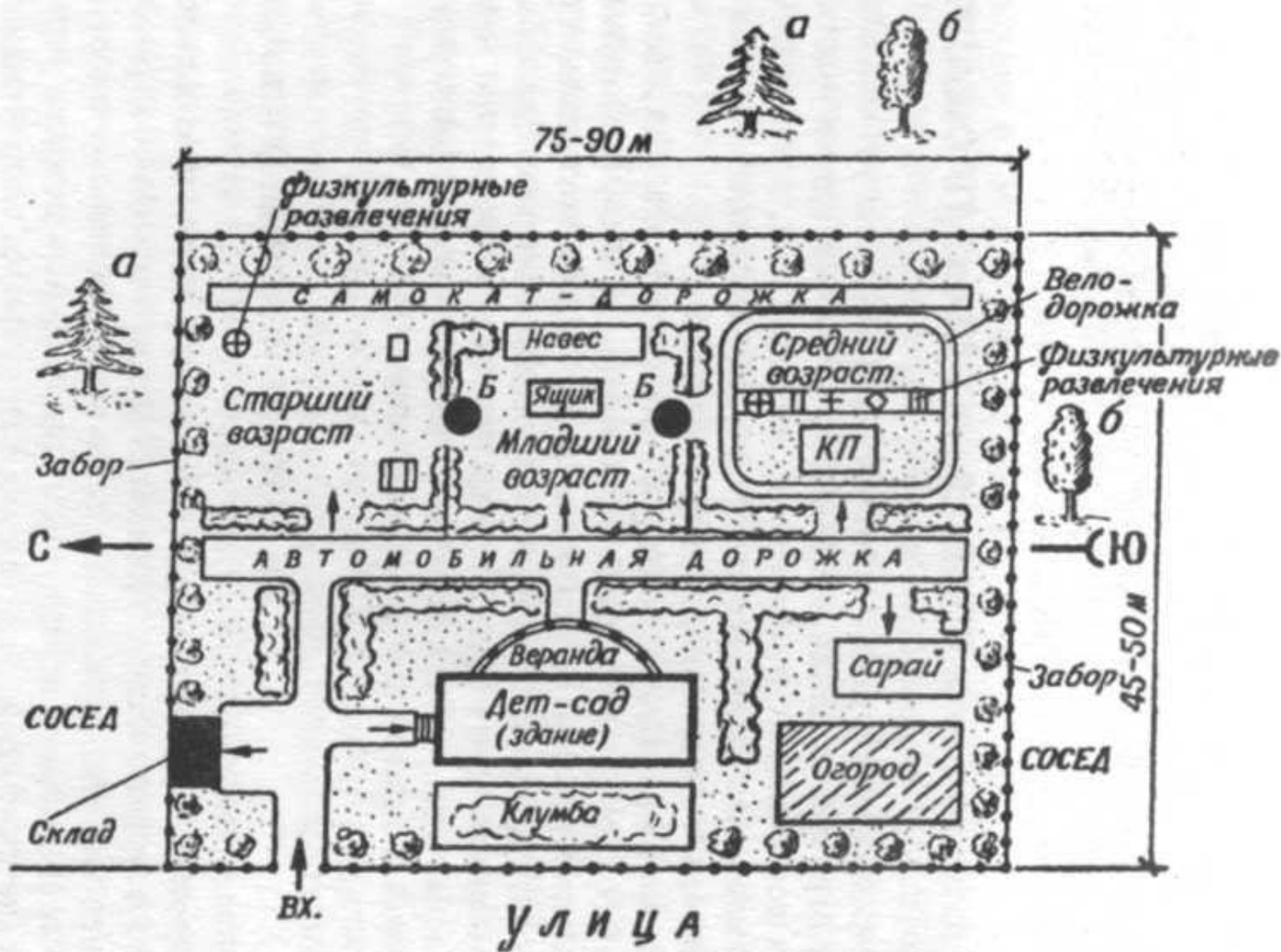
Рис. 1. Примерная схема планировки участка детского сада: а — хвойные деревья; б — лиственные деревья; Б — беседки; вх. — вход
