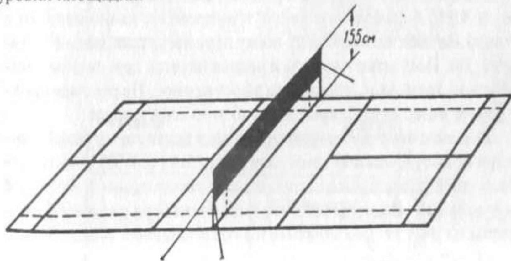
Рис. 15. Площадка для бадминтона (общий вид)
