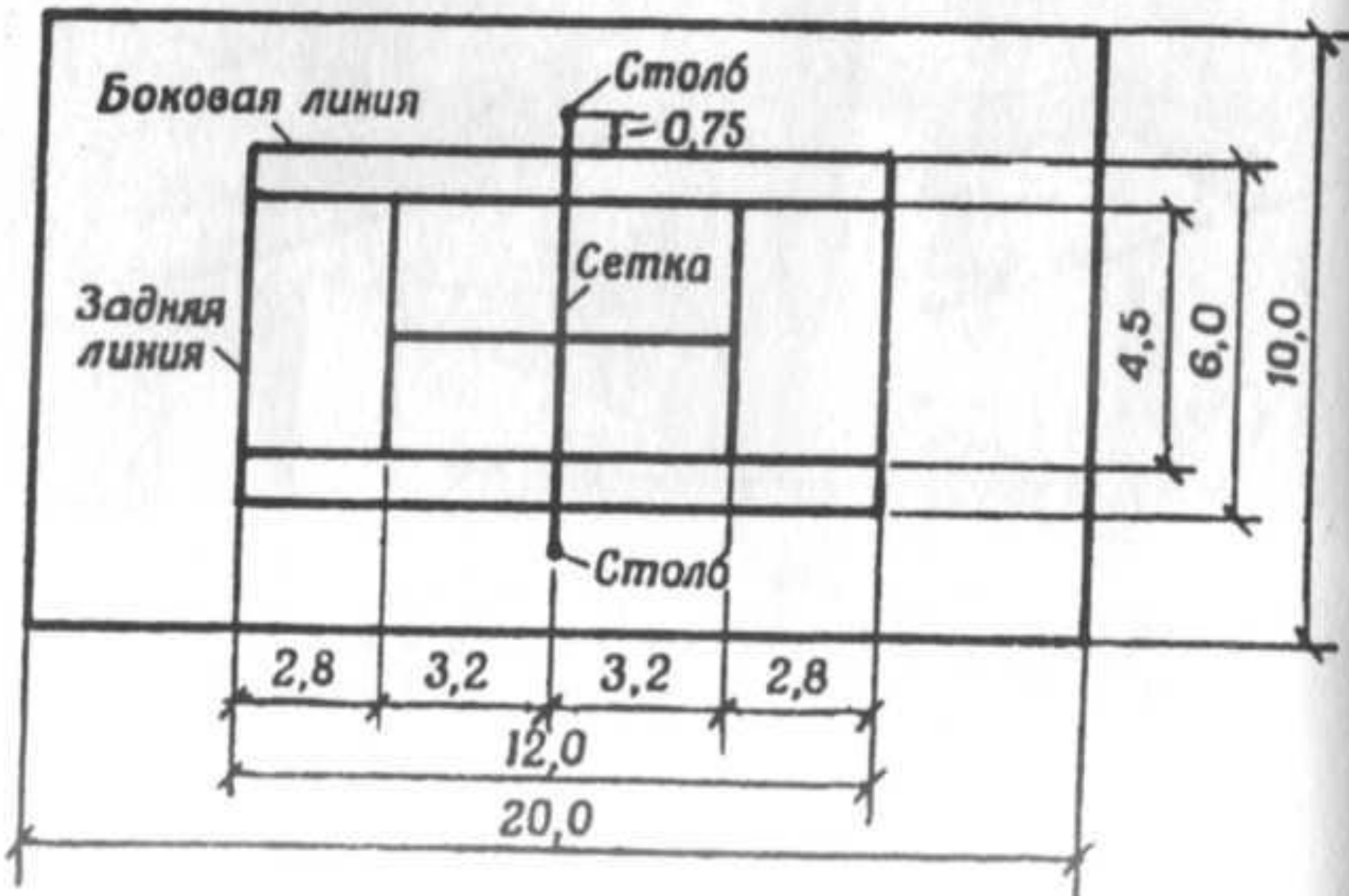
Рис. 23. Площадка для малого тенниса
