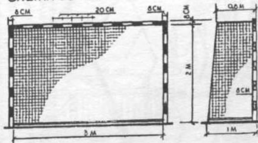
Рис. 17. Площадка для ручного мяча: а — план; б — ворота
