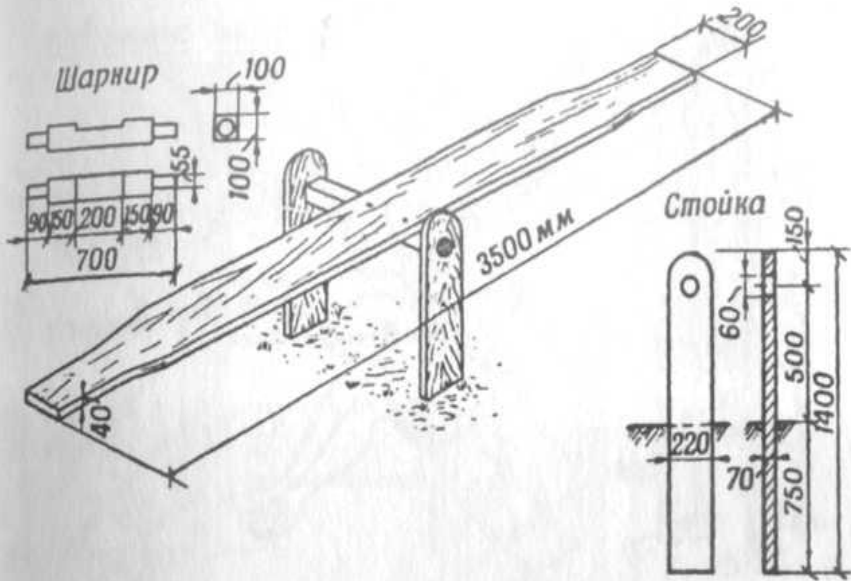
Рис. 3. Качалки простые детские (размеры в мм)
