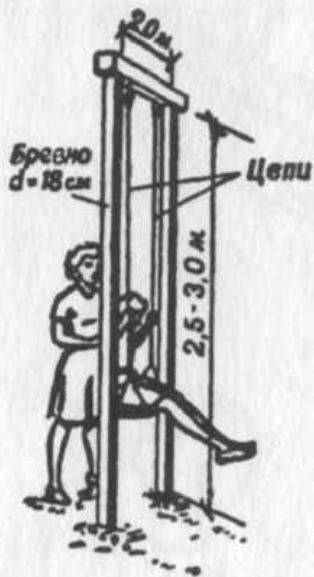
Рис. 4. Детские простые качели для детей дошкольного возраста
