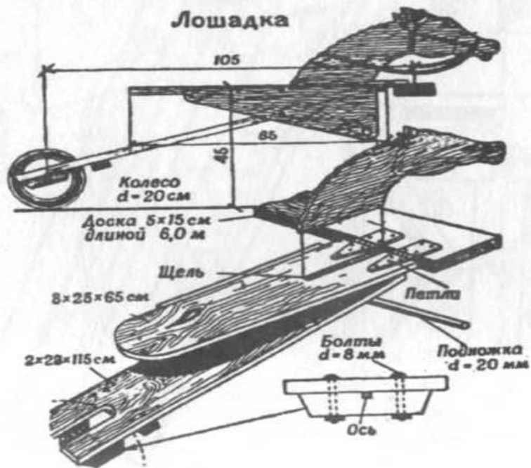
Рис. 30. Карусель с лошадками для младших школьников. Общий вид и деталь лошадки
