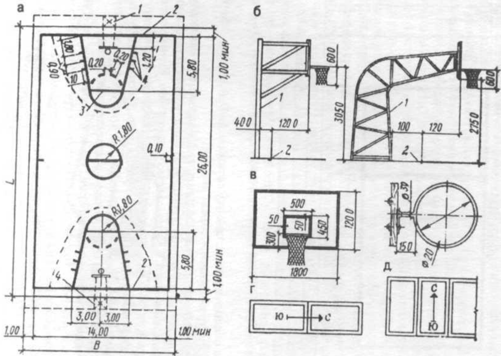
Рис. 14. Баскетбольная площадка: а — план; б — конструкция стоек; в — размеры шита, кольца
