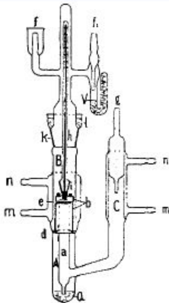
Рис. 39. Первый диффузионный насос Геде (1913 г.)
