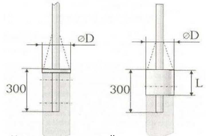
Крепление кронштейна на опору сверху
