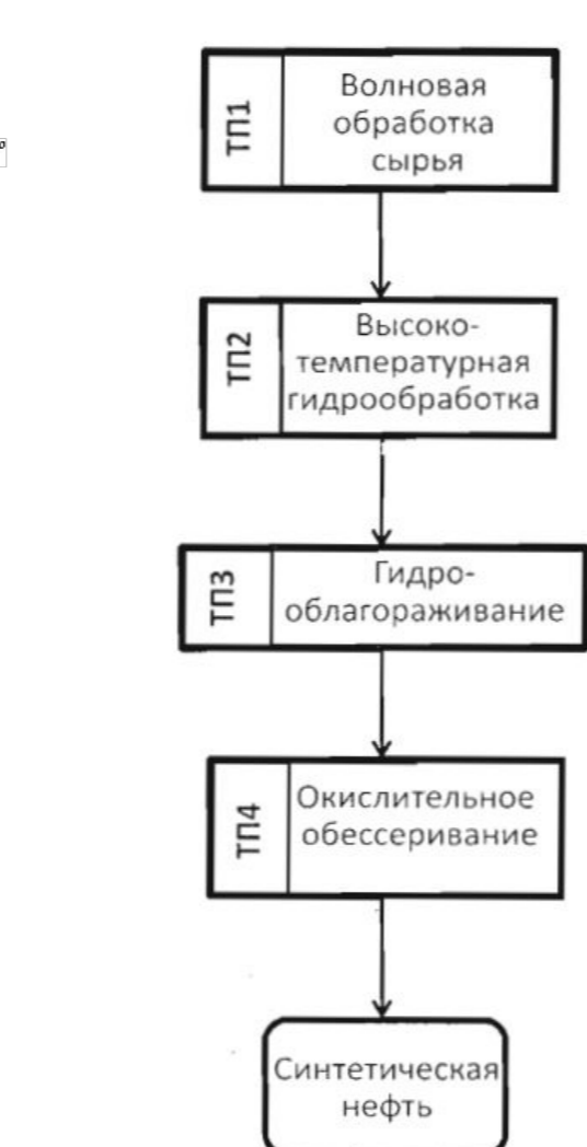
Технологическая схема процесса переработки керогенсодержащих пород в синтетическую нефть
