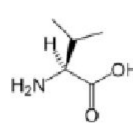
L-Leucine
