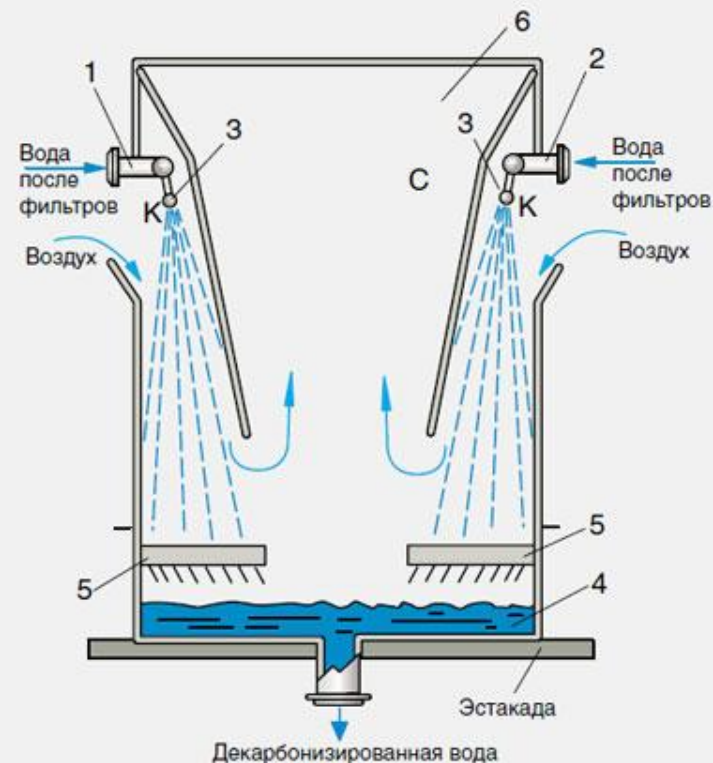
Рис. 3. Схема прямооточного распылительного двухсекционного декарбонизатора:
