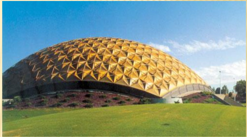
Купол Фуллера
