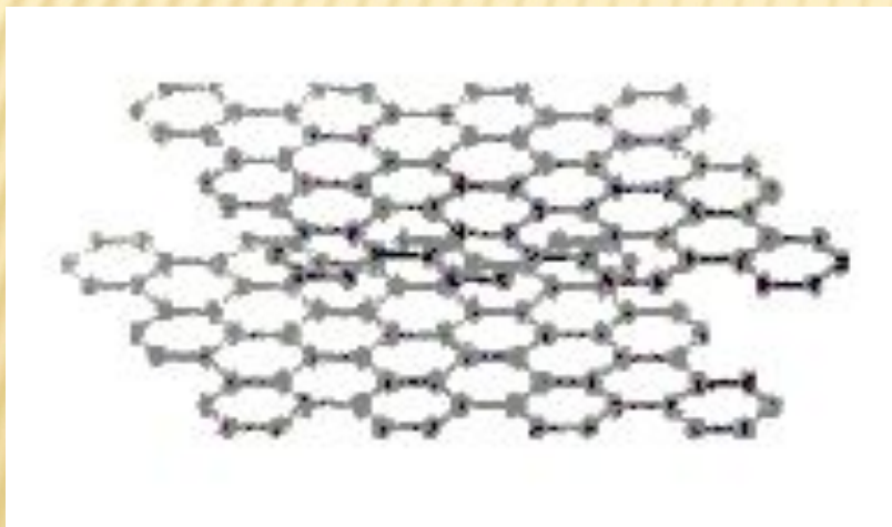
Структура графита
