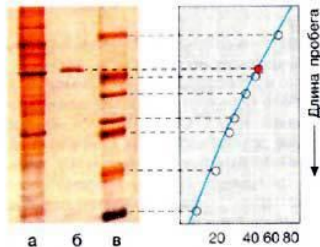
4. Определение мол. массы
