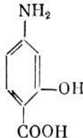
Пара-аминосалициловая кислота
