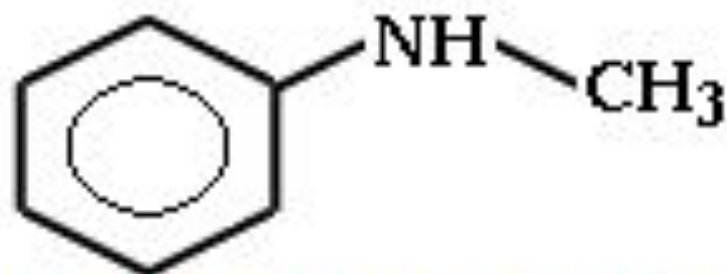
Метилфениламин
