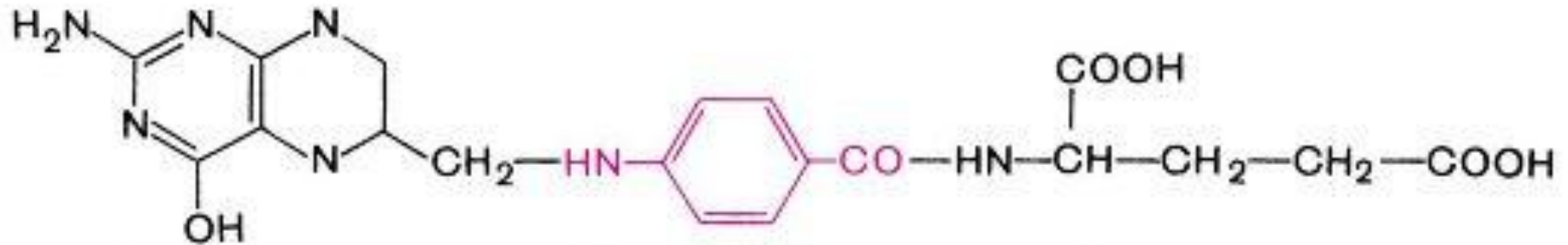
Дигидроптеридинил
