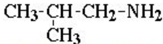
2-Метилпропанамин-1 (изобутиламин)
