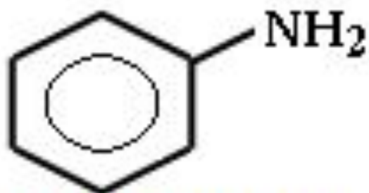
Фениламин (анилин)
