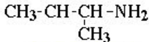
Бутанамин-2 (втор-бутиламин)
