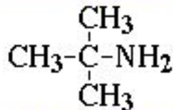
2-Метилпропанамин-2 (трет-бутиламин)
